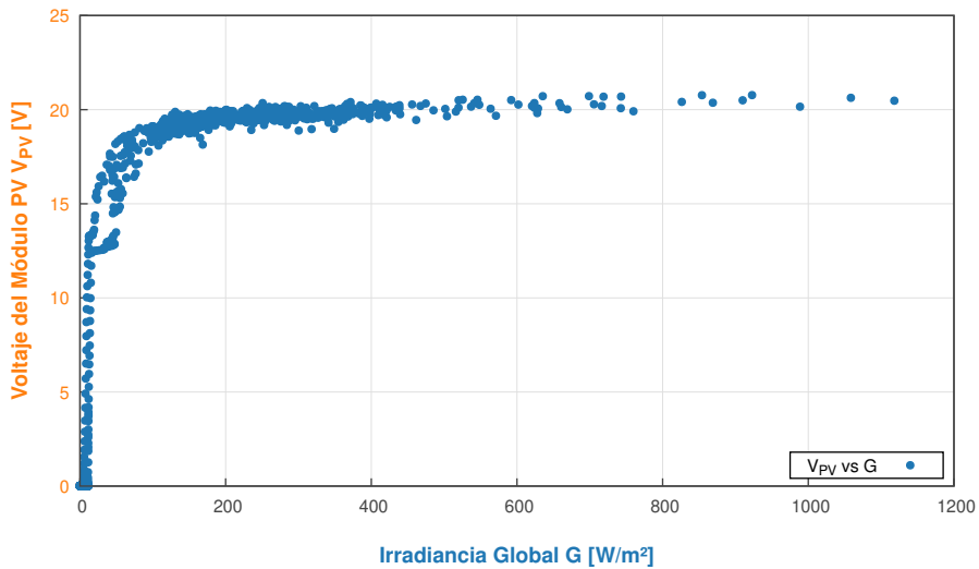
Relación entre Irradiancia Incidente y Voltaje del Módulo PV - 2026-08-13
