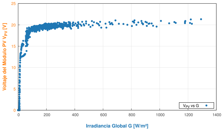
Relación entre Irradiancia Incidente y Voltaje del Módulo PV - 2026-08-14
