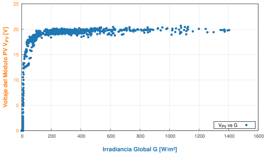
Relación entre Irradiancia Incidente y Voltaje del Módulo PV - 2026-08-15
