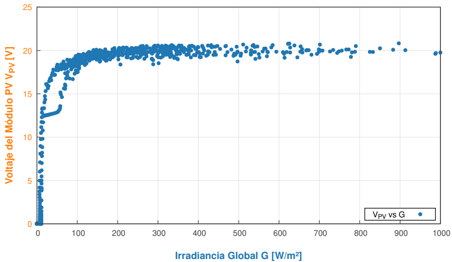
Relación entre Irradiancia Incidente y Voltaje del Módulo PV - 2026-08-16
