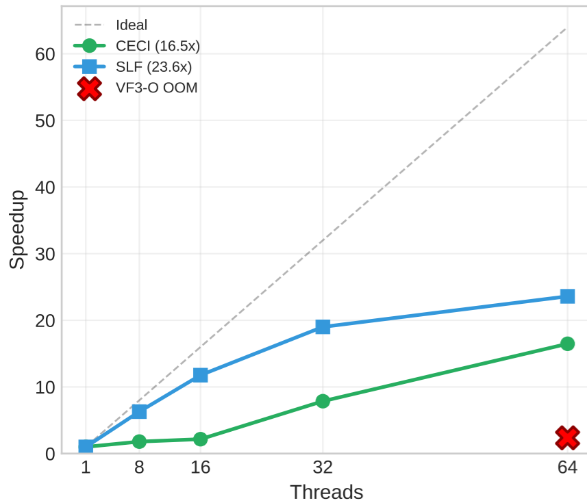
Dense 8v
