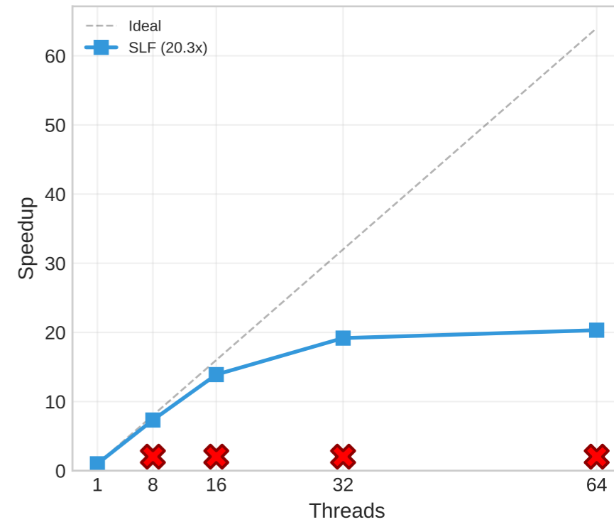
Dense 32v
