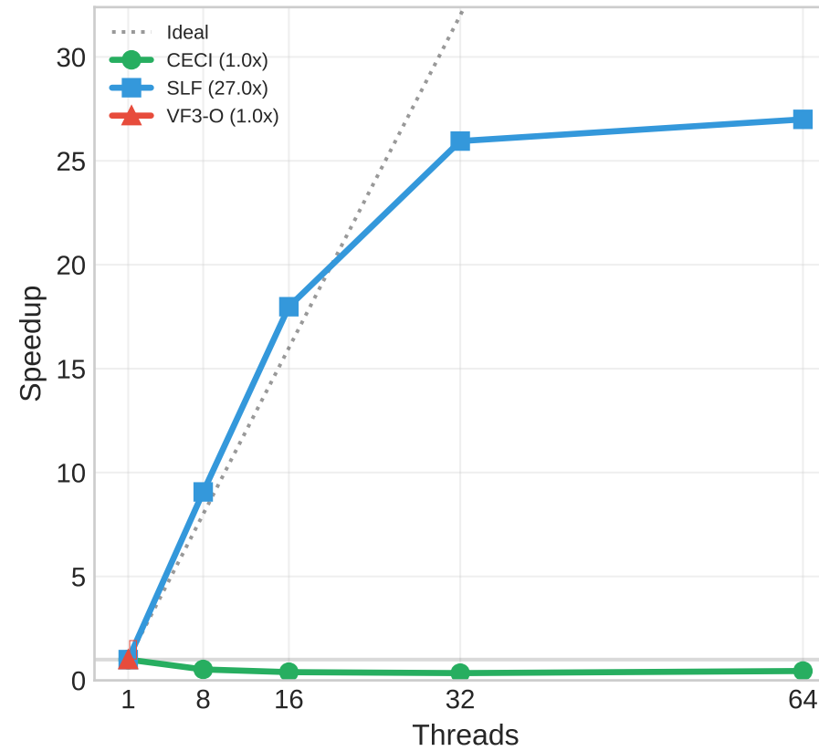
Dense 16v
