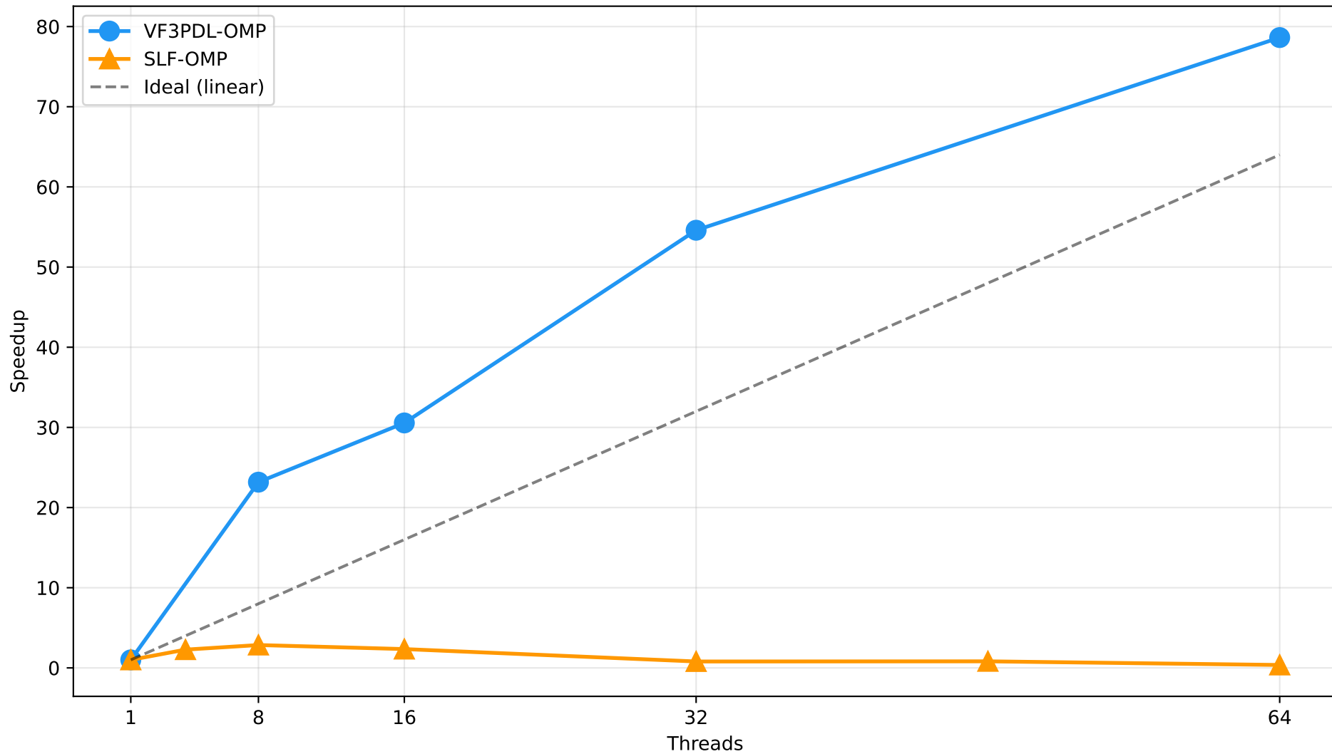
RQ1: Speedup (ENRON Sparse 8v)
