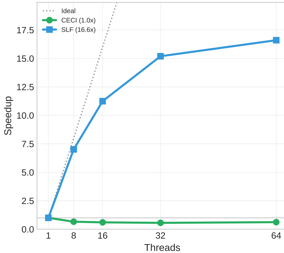
Dense 32v
