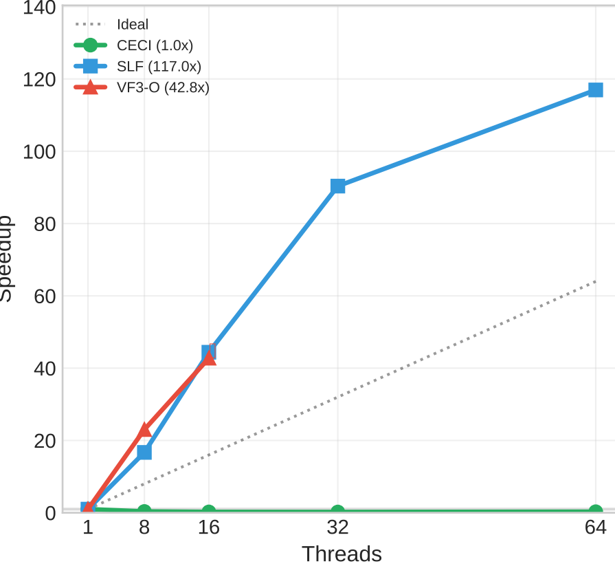
Dense 8v
