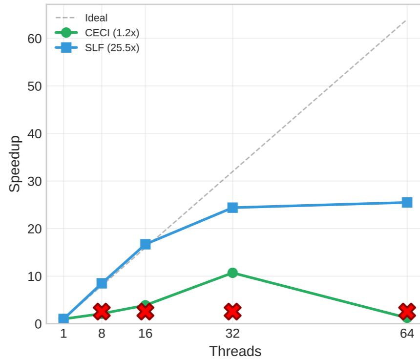
Dense 16v
