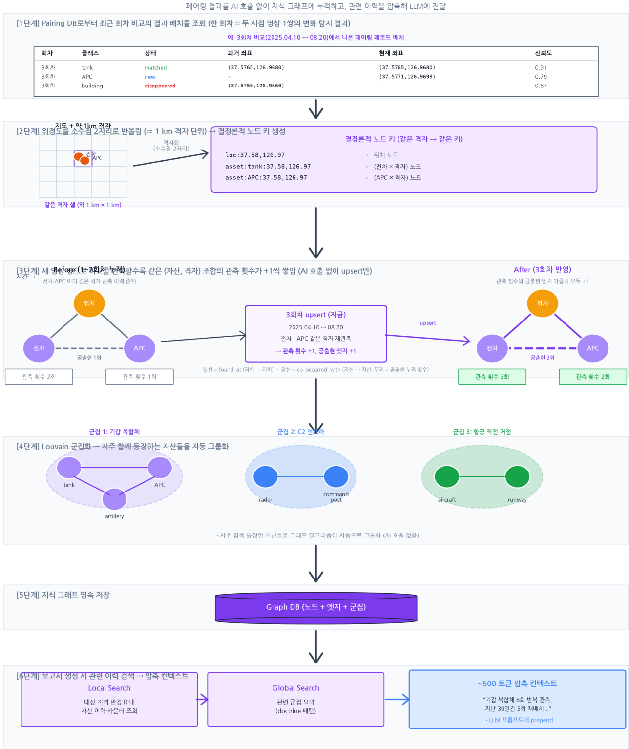
도 3. GraphRAG 기반 시공간 이력 누적 및 압축 컨텍스트 생성
