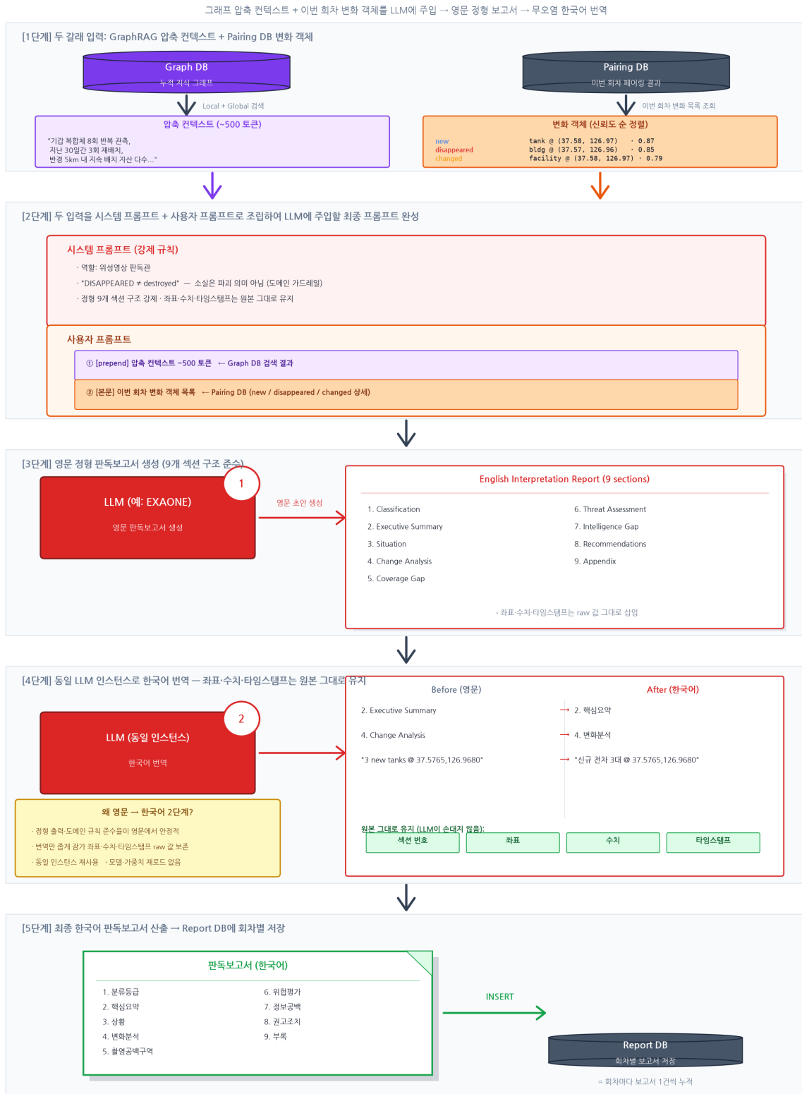
도 4. 판독보고서 자율 생성
