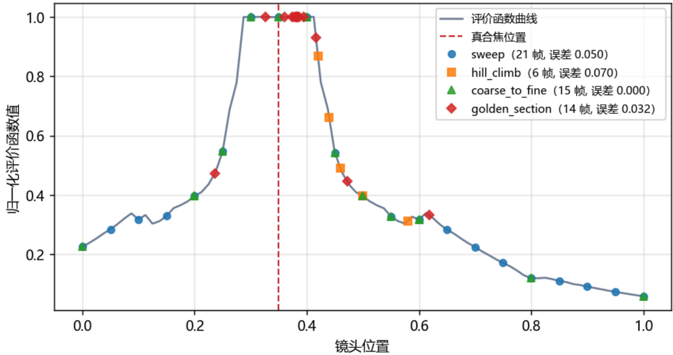
搜索策略：帧数 vs 定位精度 (爬山法帧数最少，但没有利用单峰性，精度最差)
