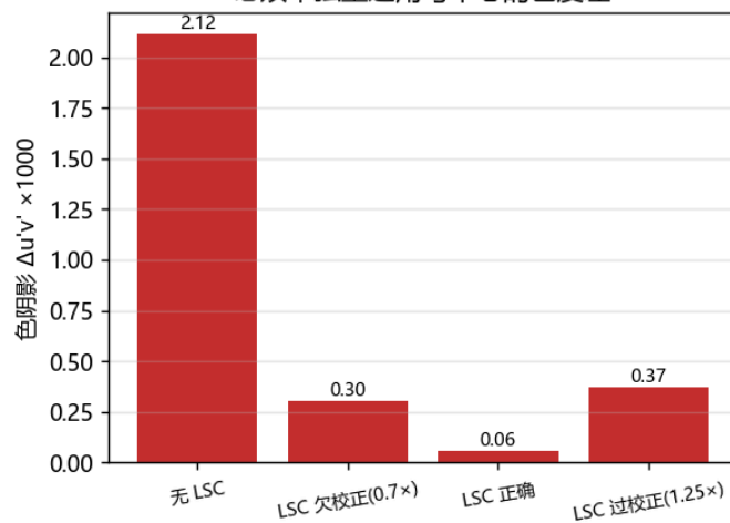
色阴影：只看亮度均匀度是看不出来的 必须单独量边角与中心的色度差
