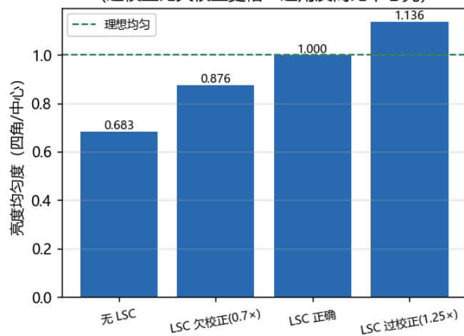
LSC 校正准 / 欠 / 过 (过校正比欠校正更糟：边角反而比中心亮)
