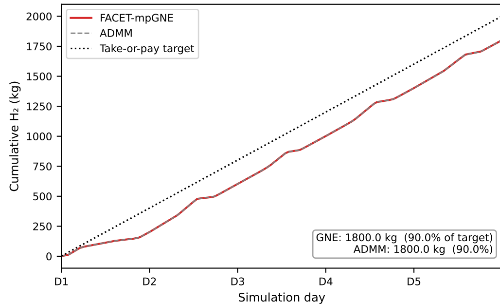
PEM H 2 production
