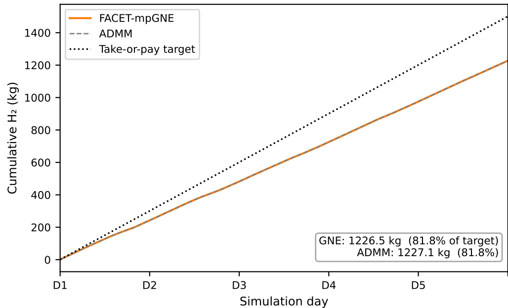
Alk H 2 production
