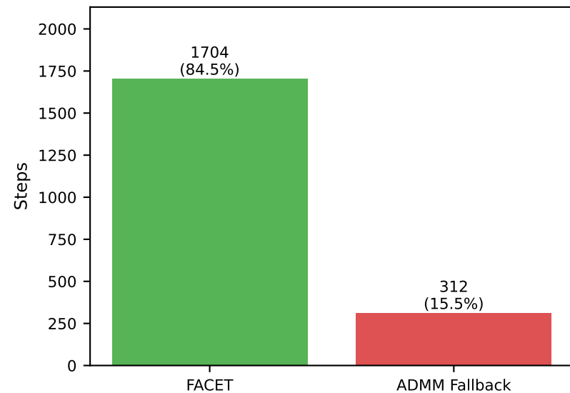
FACET solve-path per step
