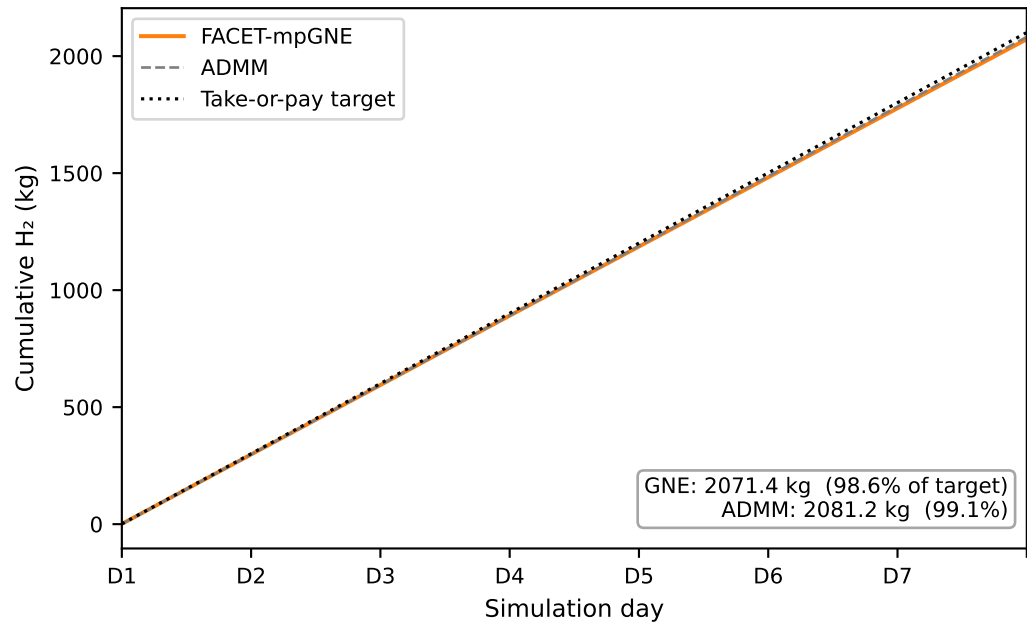
Alk H 2 production
