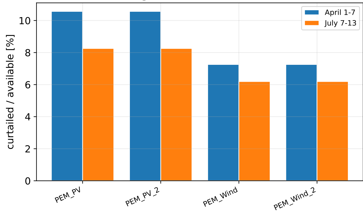
Per-agent curtailment fraction
