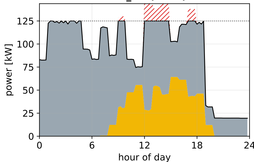
PEM_PV (solar)
