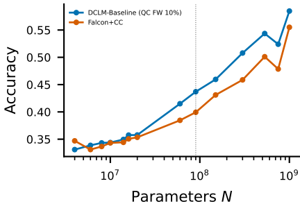
olmes_10_macro_avg
