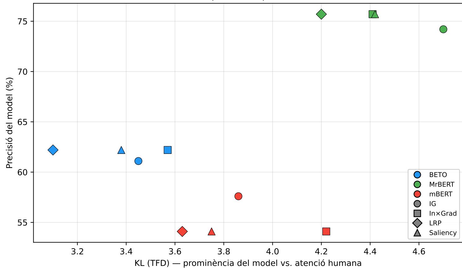
Dispersió KL-precisió
