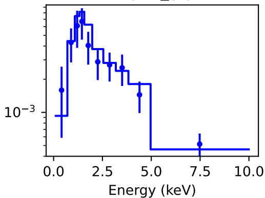
mos2spec_grp.fits
