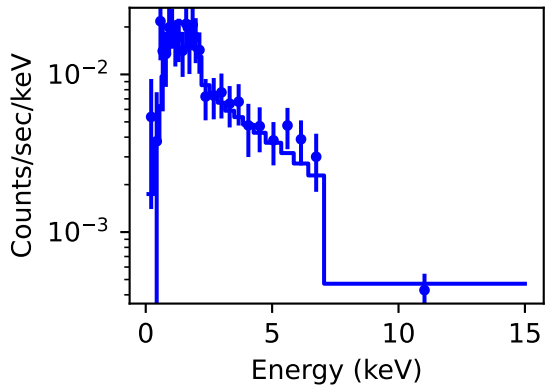
pnspec_grp.fits
