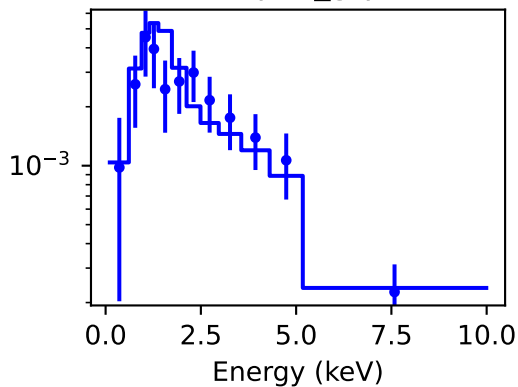
mos2spec_grp.fits
