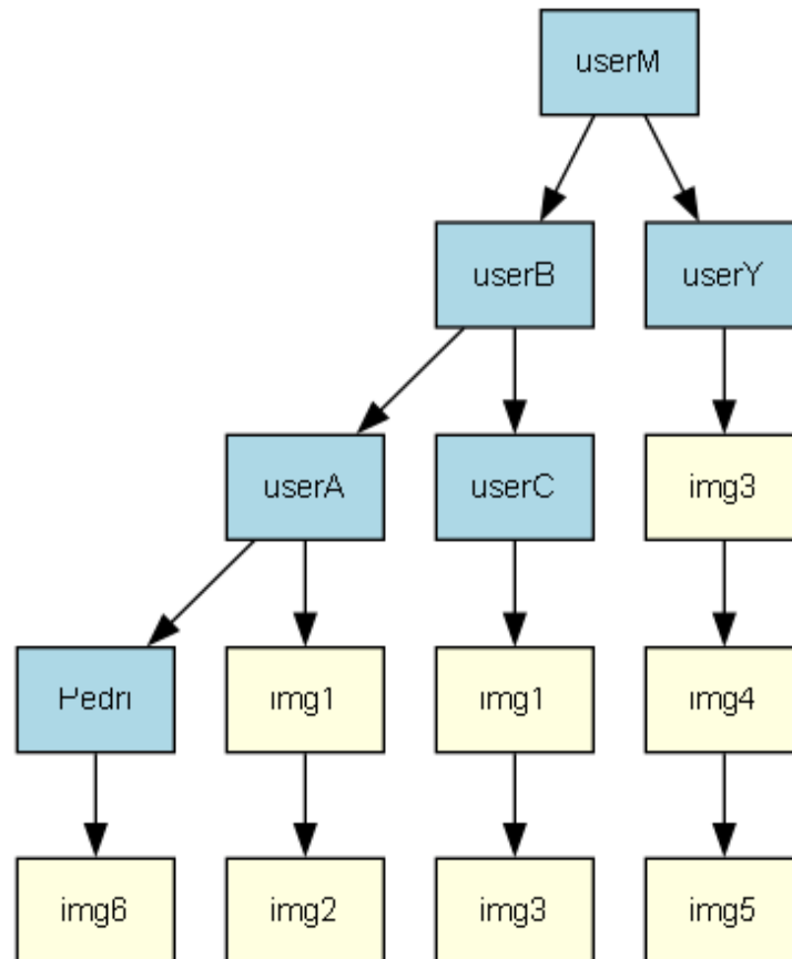
Fig. 3.4 — ABB de Usuarios con los datos de ejemplo
