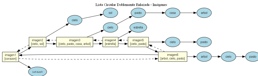
Fig. 3.3 — Lista Circular Doblemente Enlazada de Imágenes
