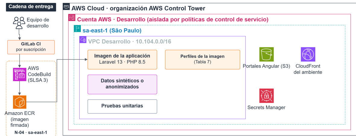
Figura 3 Ambiente de Desarrollo
