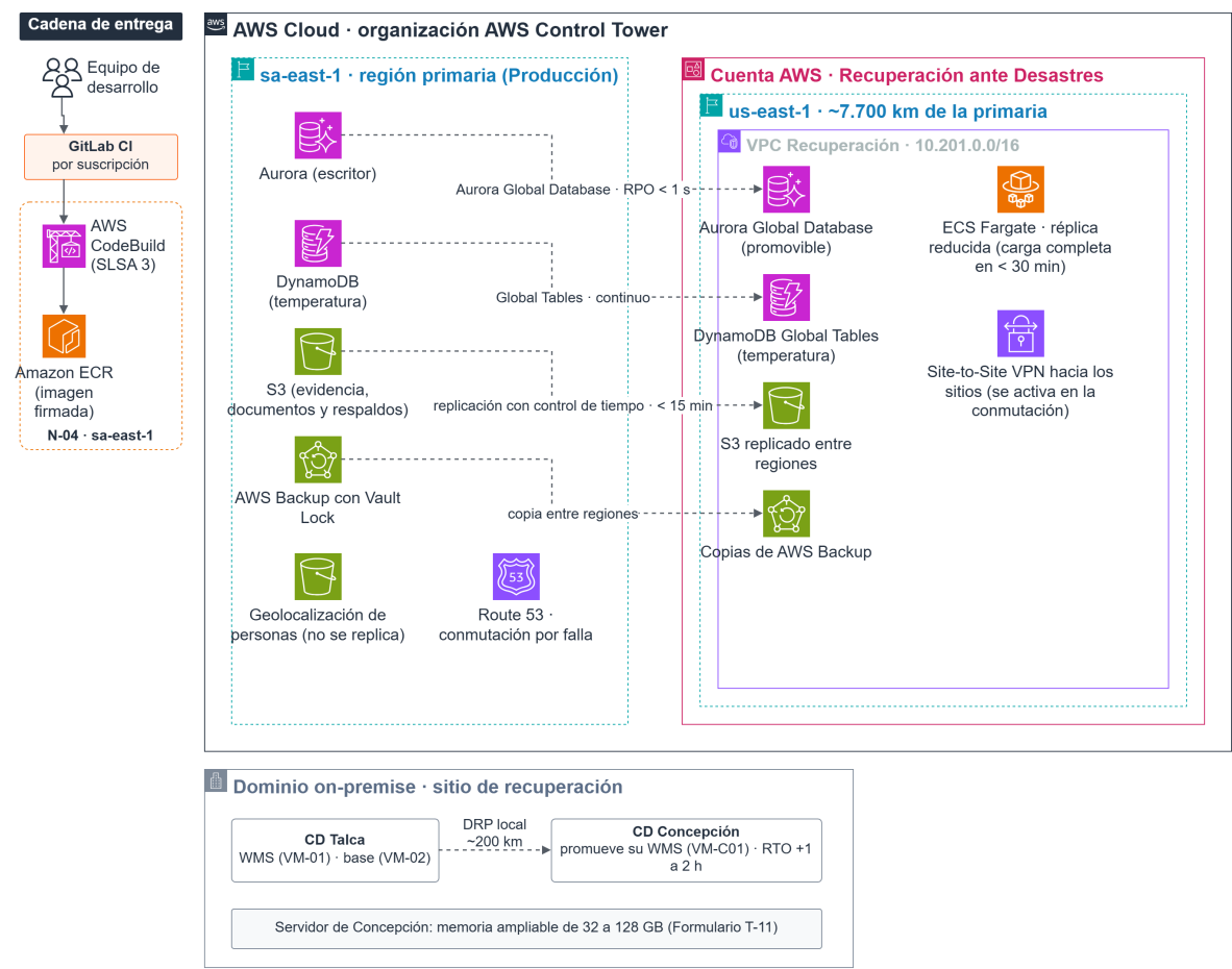
Figura 7 Ambiente de Recuperación ante Desastres
