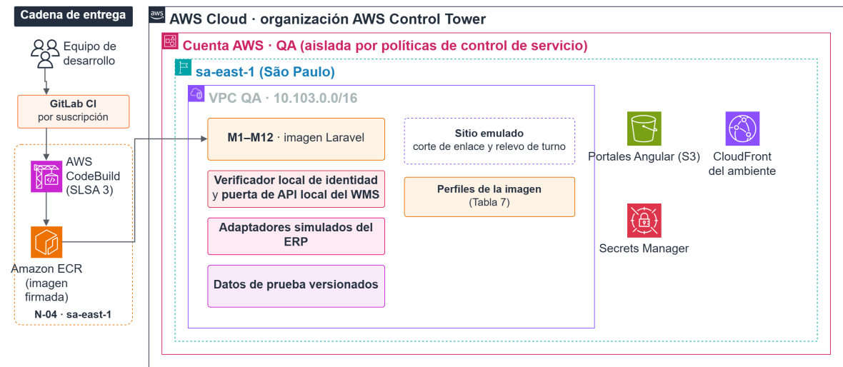
Figura 4 Ambiente de QA
