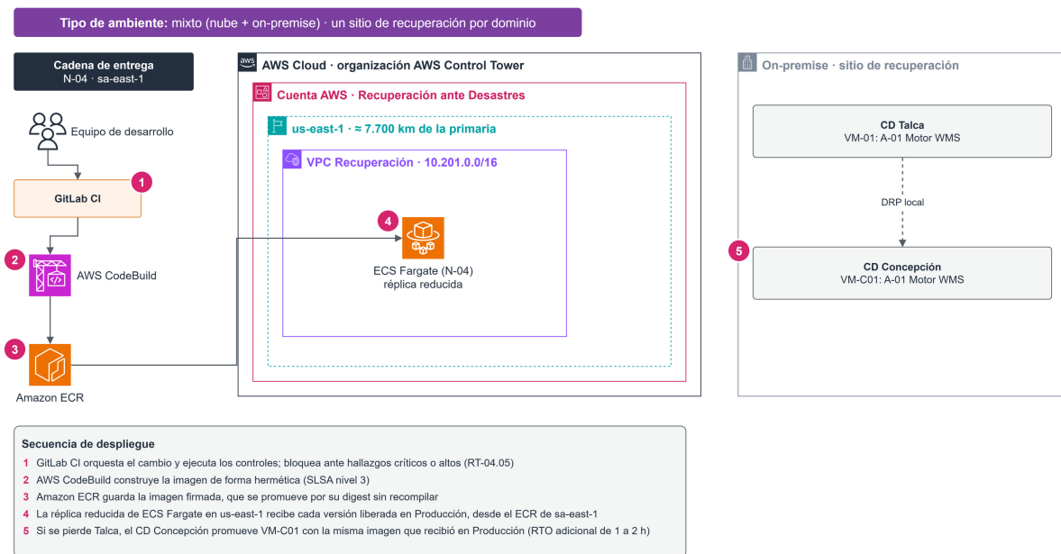
Figura 9 Ambiente de Recuperación ante Desastres
