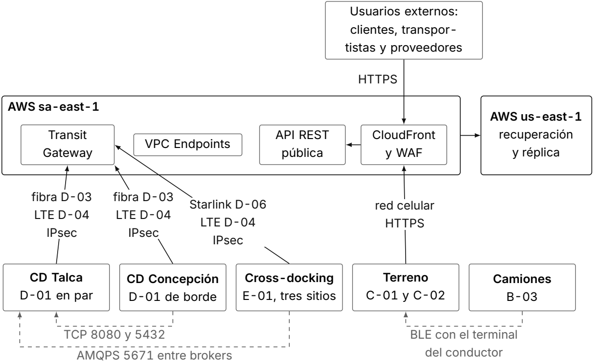
Figura 10 Conexiones entre los sitios, el terreno y la nube Fuente: elaboración propia.
