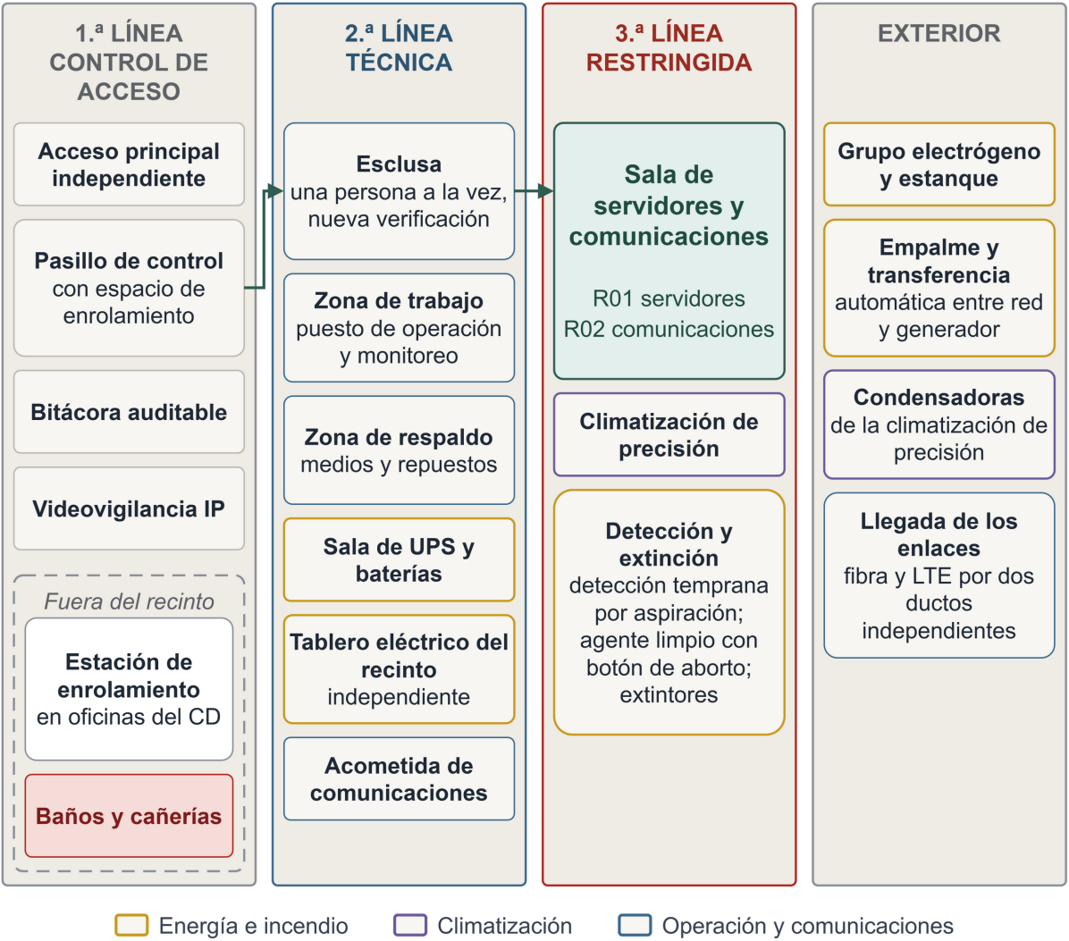
Figura 15 Distribución interna del recinto técnico del CD Talca por zonas y líneas de acceso Fuente: elaboración propia.
