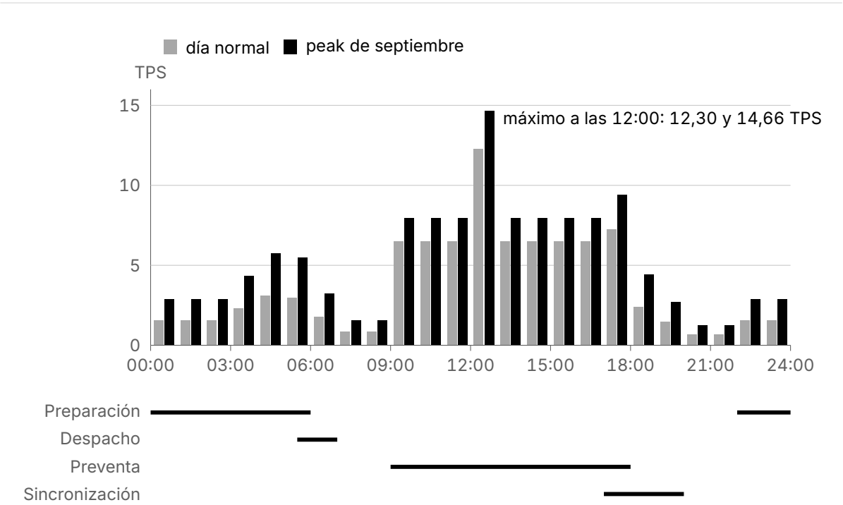
Figura 12 Tasas totales por hora en régimen normal y en septiembre. Fuente: elaboración propia.
