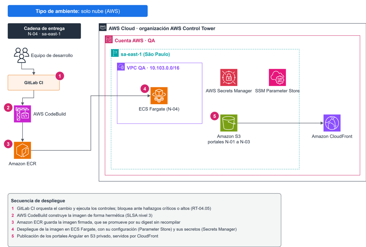
Figura 6 Ambiente de QA
