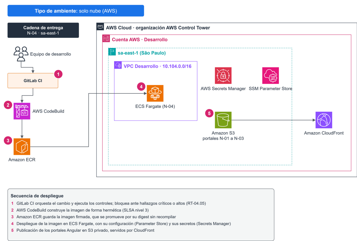
Figura 5 Ambiente de Desarrollo
