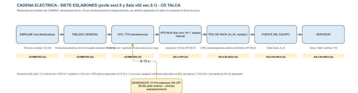
Figura 4 Cadena eléctrica del recinto: acometida, transferencia automática, generación autónoma, alimentación ininterrumpida y distribución A/B por gabinete
