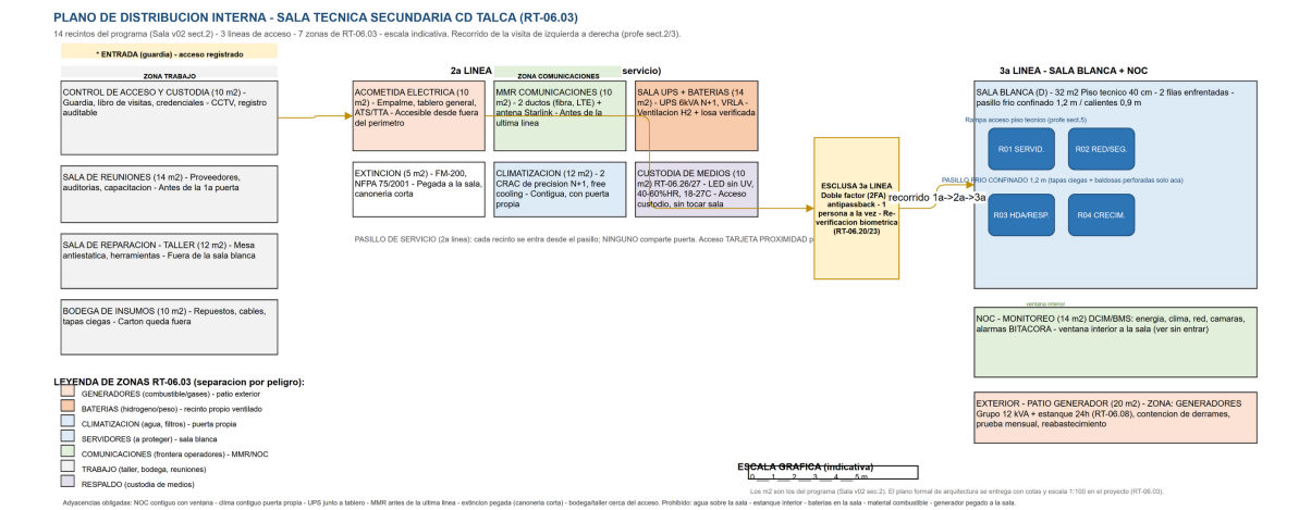
Figura 3 Plano de distribución interna del recinto técnico, con la separación de las zonas de generador, baterías, climatización, servidores, comunicaciones y custodia de medios
