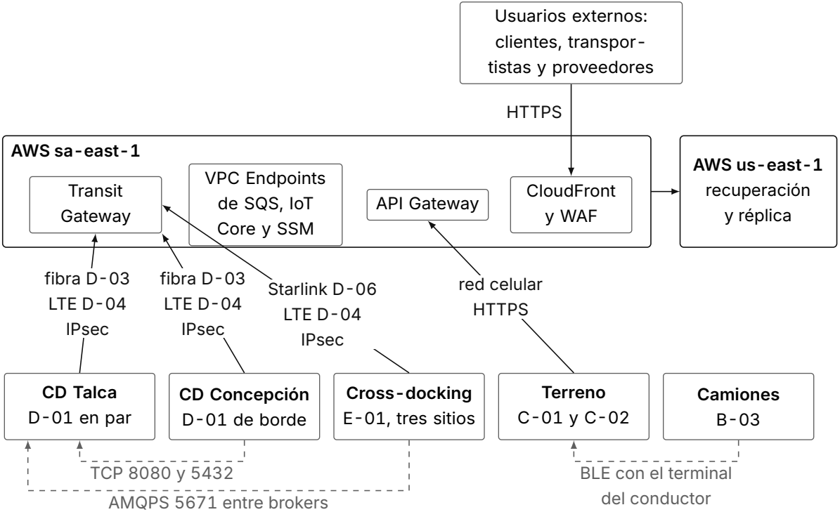
Figura 2 Conexiones entre los sitios, el terreno y la nube Fuente: elaboración propia.
