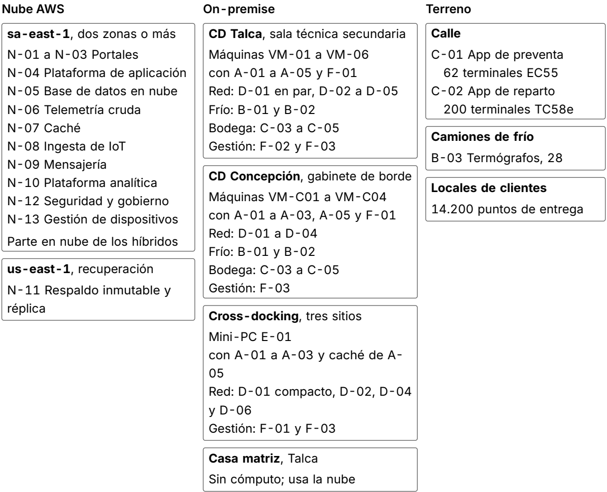
Figura 1 Ubicación de los componentes por dominio y por sitio Fuente: elaboración propia a partir del catálogo de componentes de la arquitectura lógica y de la volumetría del caso (Caso, Tabla 14.1).
