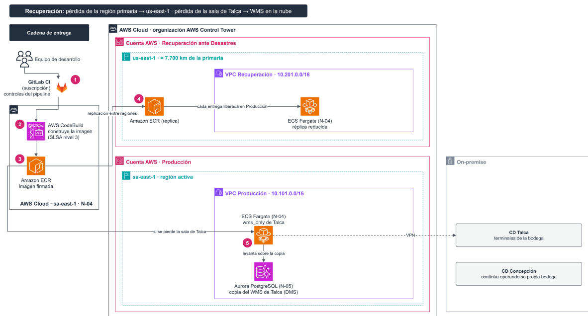
Figura 24 Ambiente de Recuperación ante Desastres
