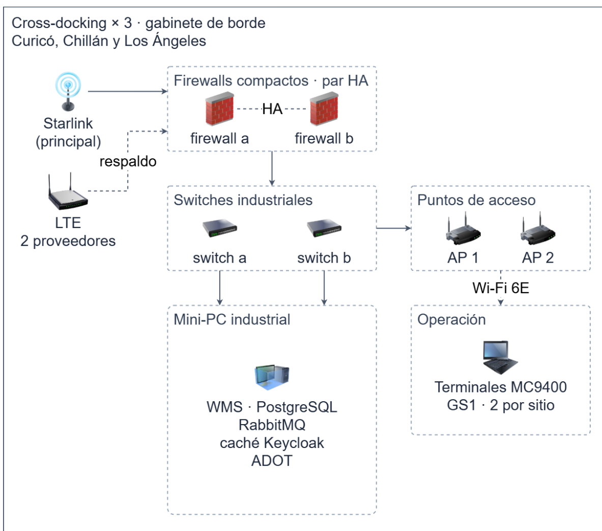
Figura 16 Gabinete de borde de las plataformas de cross-docking
