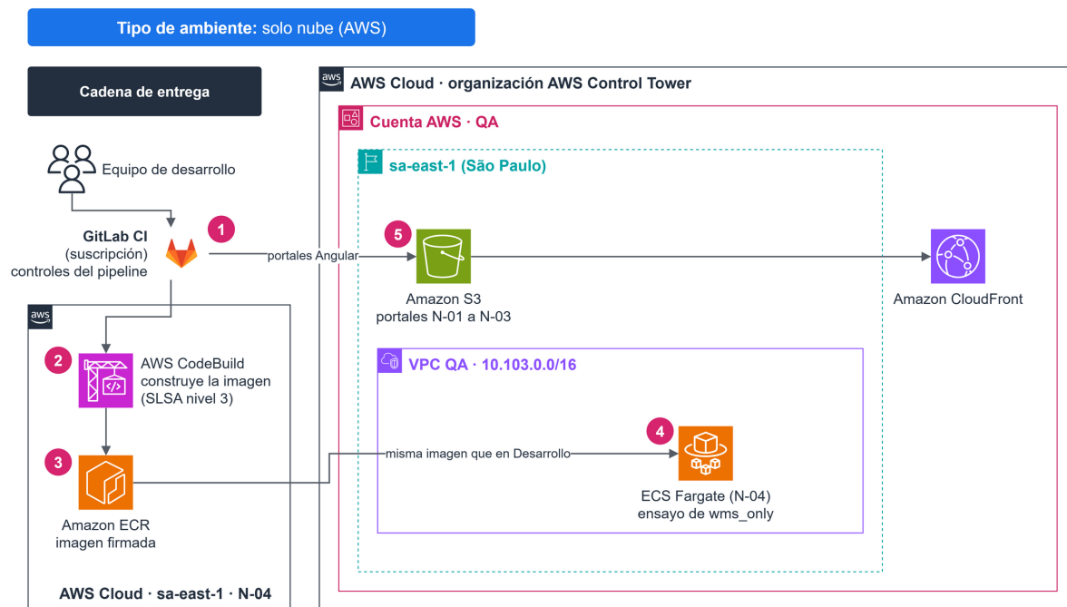
Figura 21 Ambiente de QA
