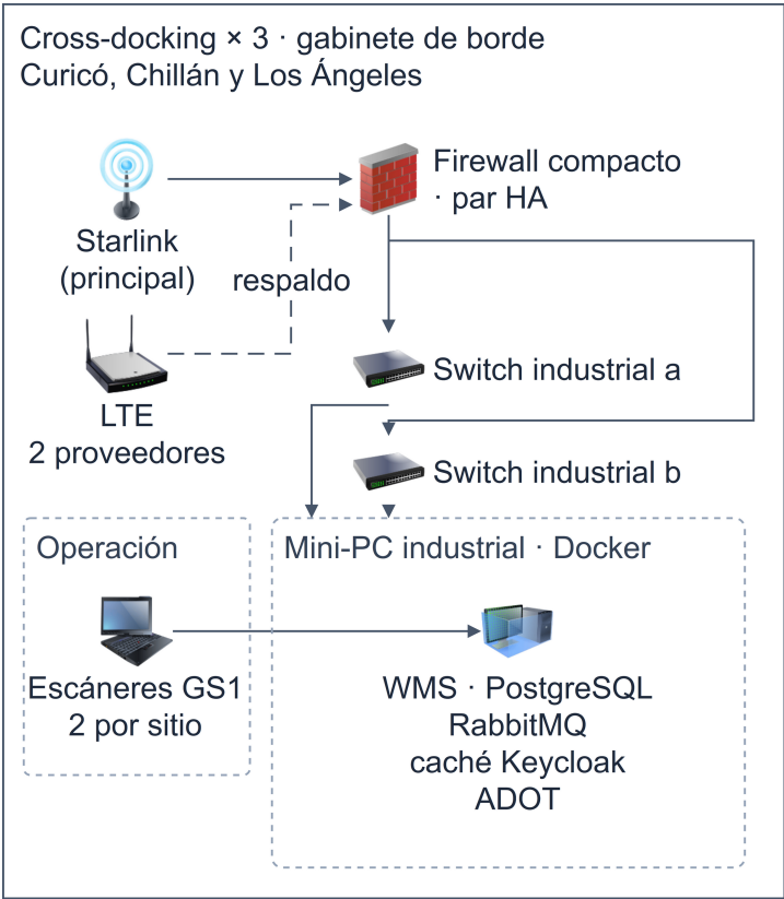
Figura 16 Gabinete de borde de las plataformas de cross-docking Fuente: elaboración propia.
