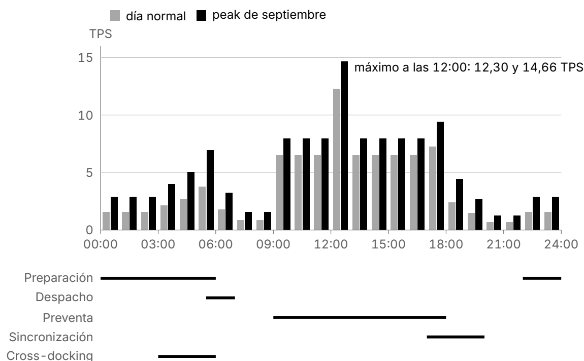
Figura 27 Tasas totales por hora en régimen normal y en septiembre.
