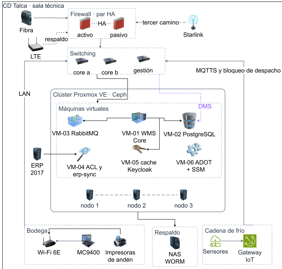
Figura 28 Arquitectura física del sitio on-premise del CD Talca
