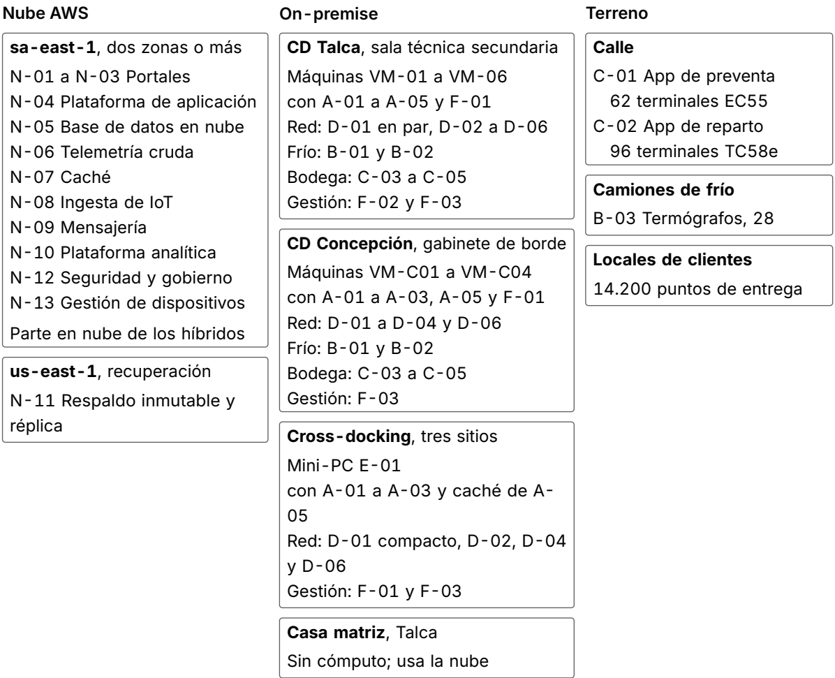
Figura 18 Ubicación de los componentes por dominio y por sitio Fuente: elaboración propia.
