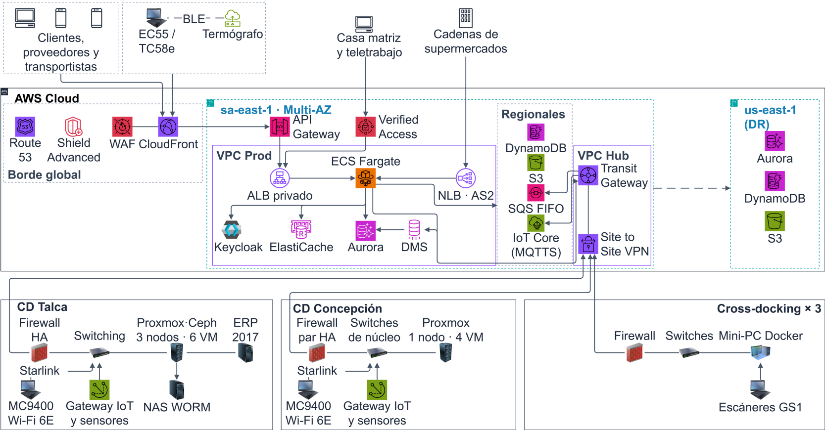
Figura 15 Vista general de la arquitectura física híbrida Fuente: elaboración propia.
