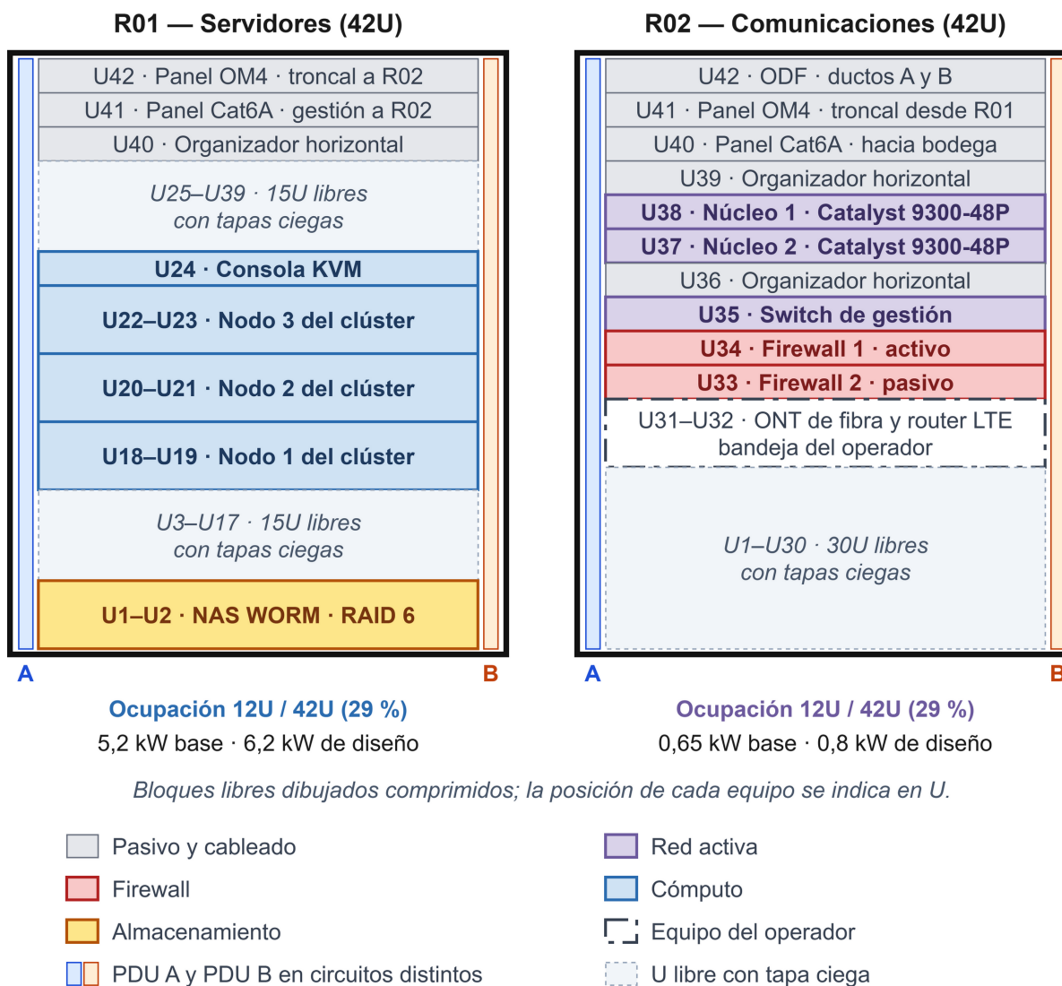
Figura 29 Distribución de U y ocupación proyectada de los racks del CD Talca
