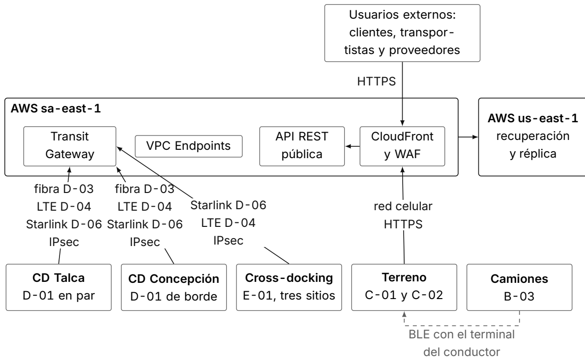
Figura 25 Conexiones entre los sitios, el terreno y la nube
