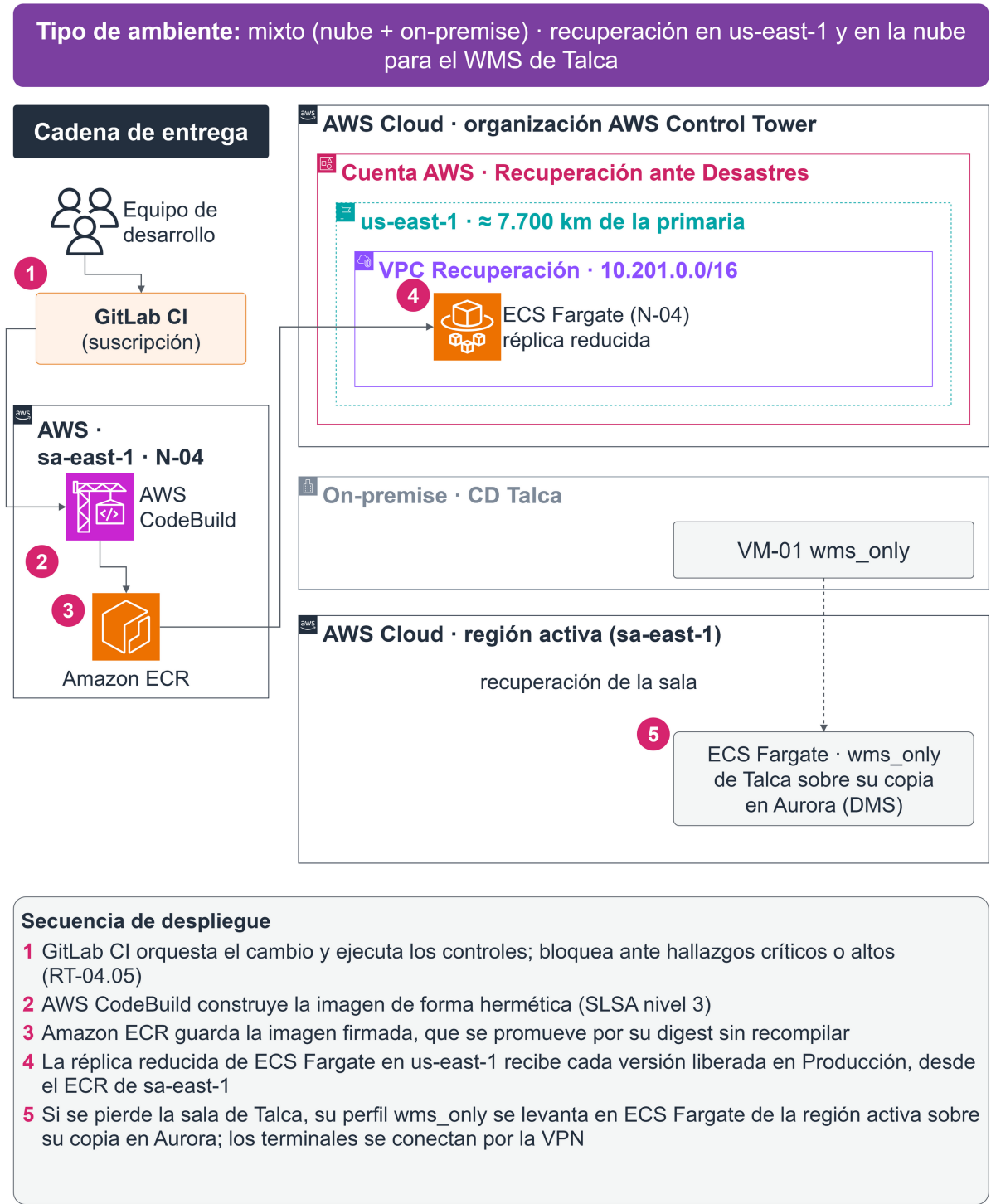
Figura 24 Ambiente de Recuperación ante Desastres
