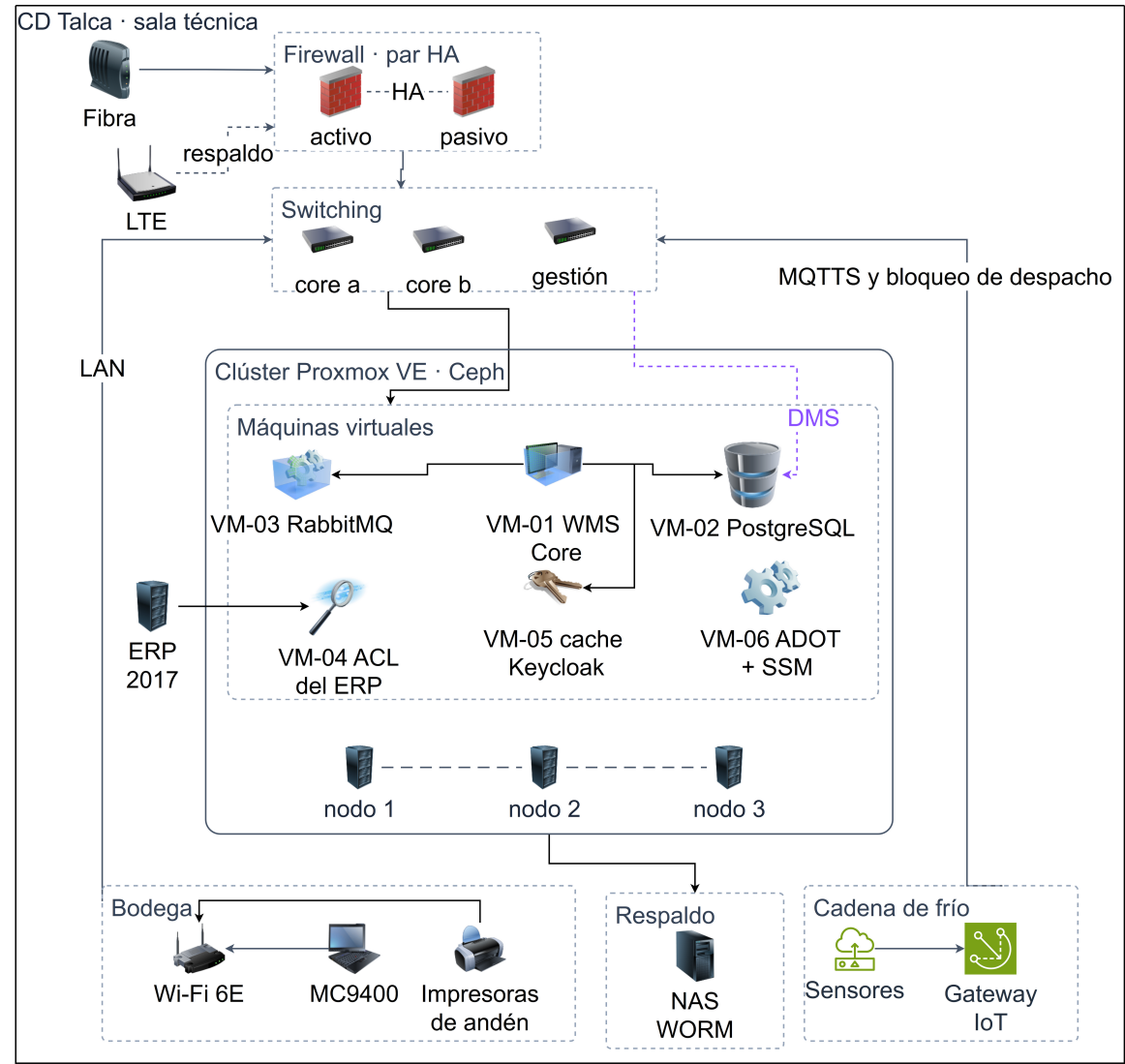
Figura 8 Arquitectura física del sitio on-premise del CD Talca Fuente: elaboración propia.
