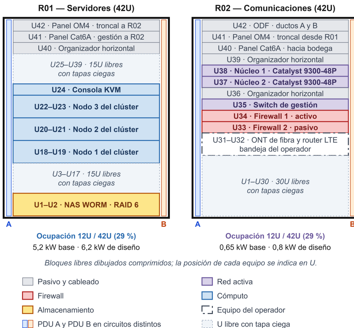
Figura 9 Distribución de U y ocupación proyectada de los racks del CD Talca
