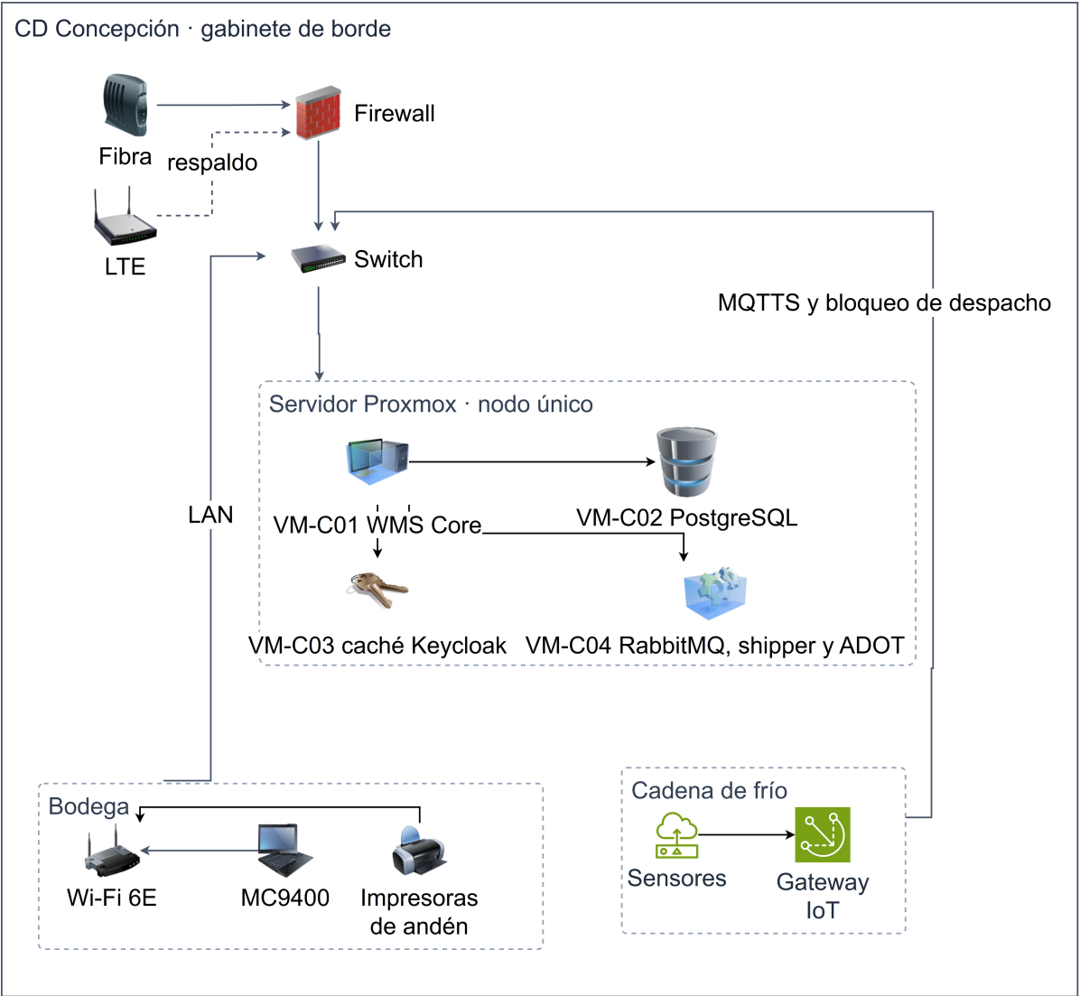
Figura 11 Gabinete de borde del CD Concepción
