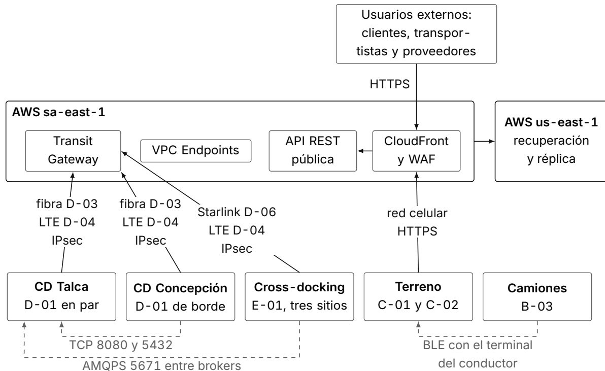
Figura 5 Conexiones entre los sitios, el terreno y la nube
