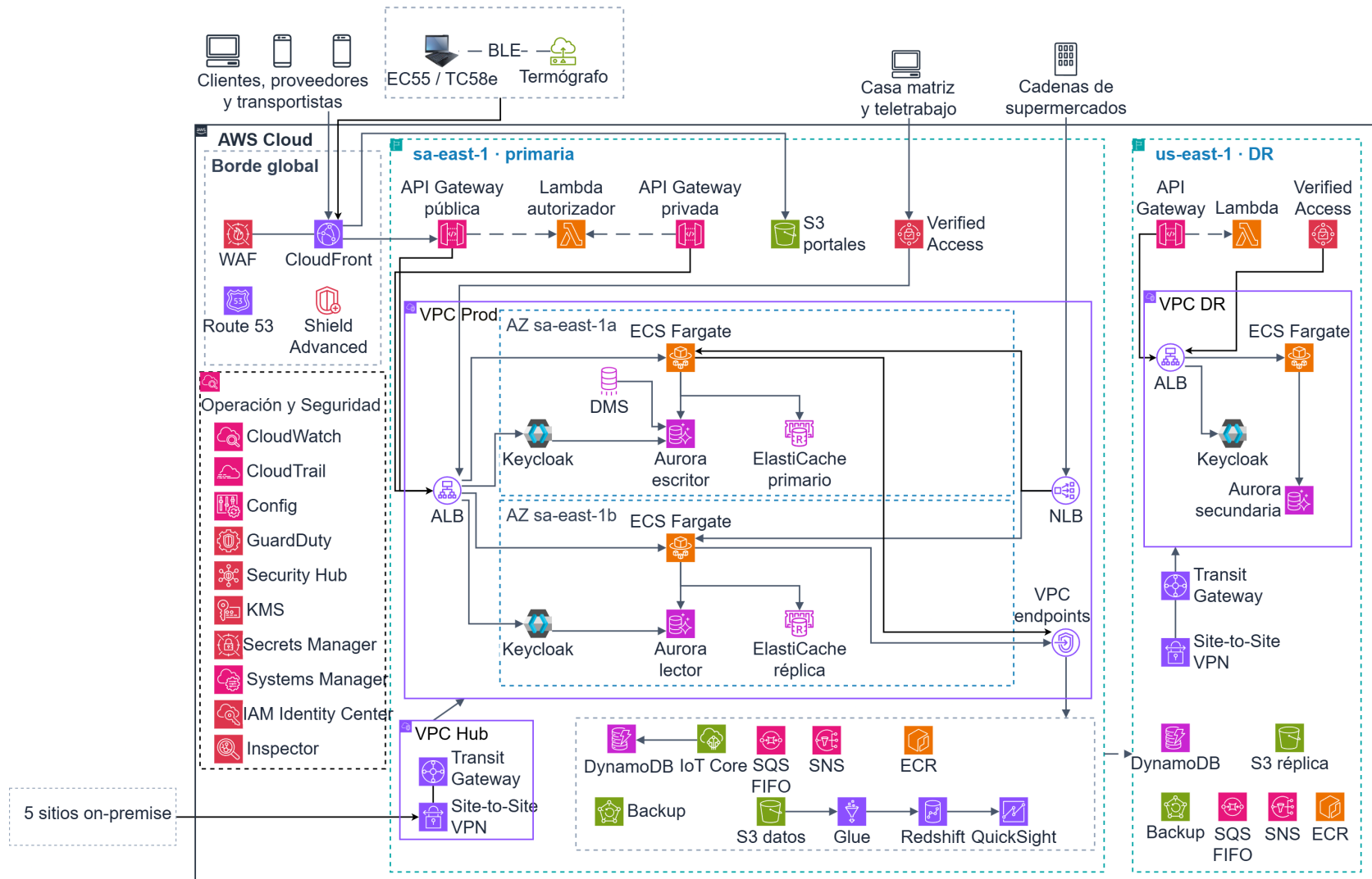
Figura 19 Topología de los servicios en AWS: región primaria sa-east-1 y región de recuperación us-east-1 Fuente: elaboración propia.
