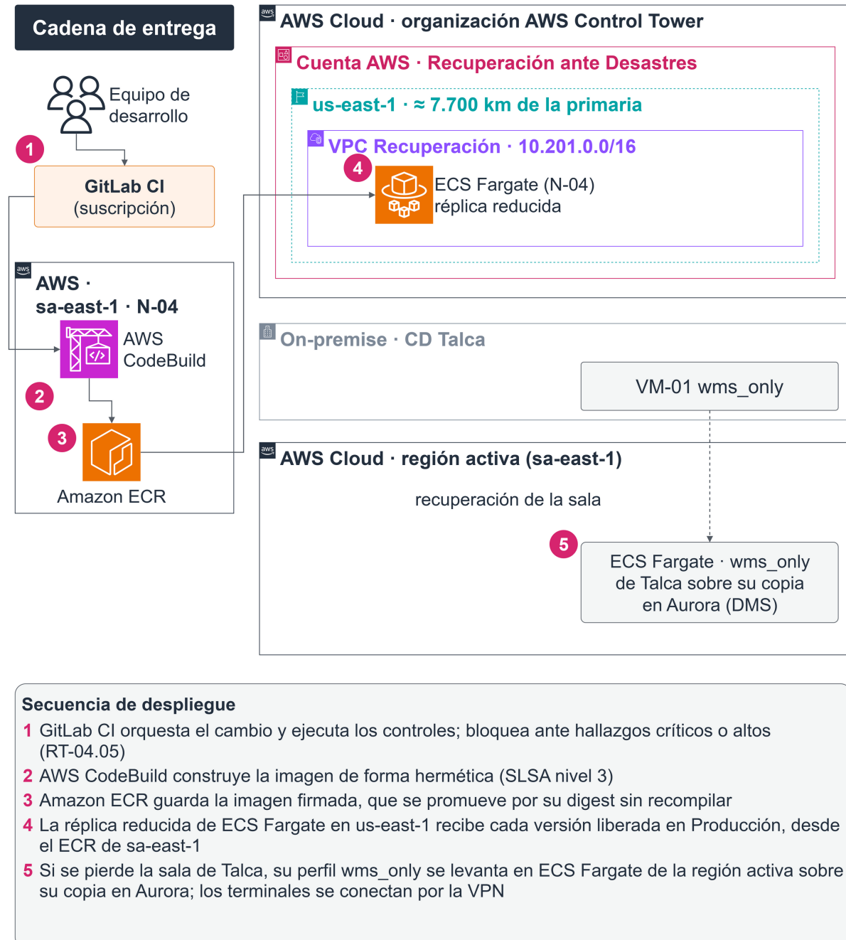
Figura 24 Ambiente de Recuperación ante Desastres
