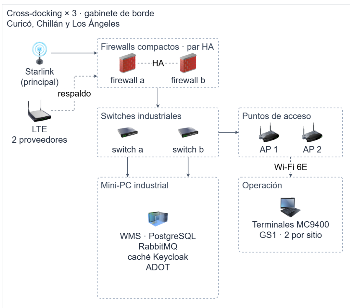
Figura 16 Gabinete de borde de las plataformas de cross-docking Fuente: elaboración propia.
