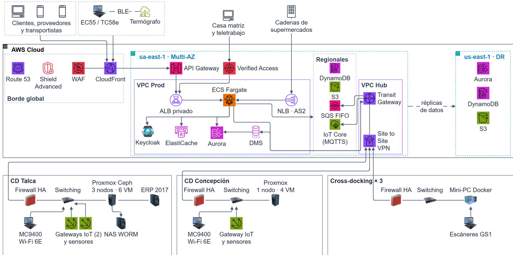
Figura 15 Vista general de la arquitectura física híbrida Fuente: elaboración propia.
