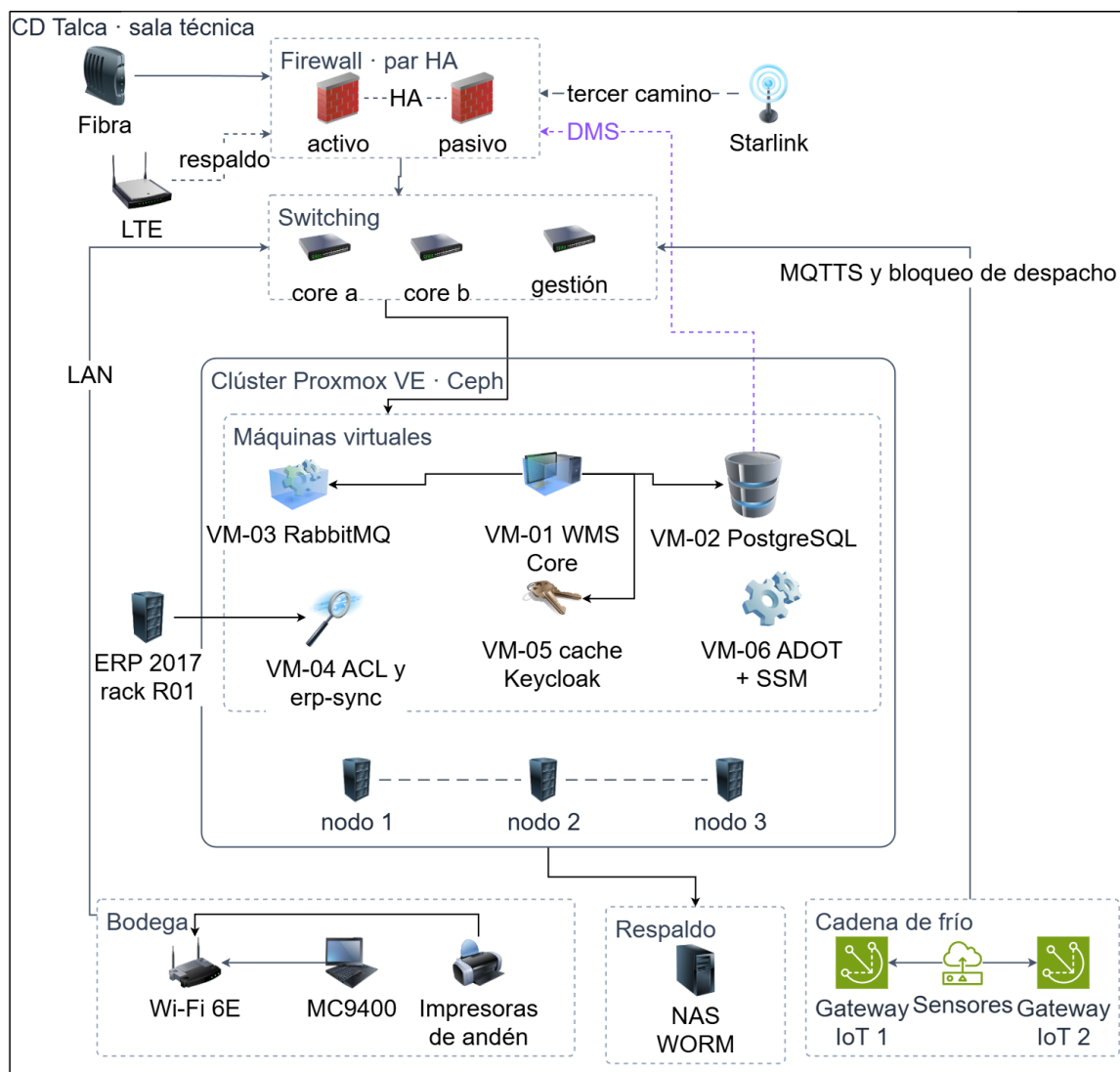
Figura 25 Arquitectura física del sitio on-premise del CD Talca
