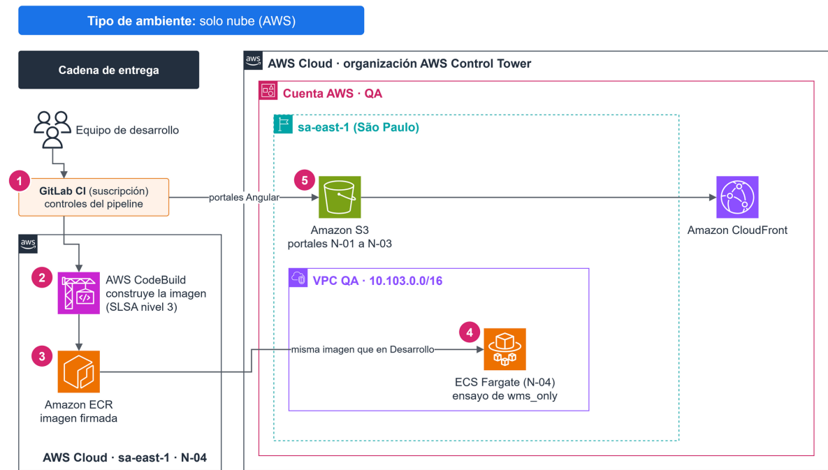
Figura 6 Ambiente de QA
