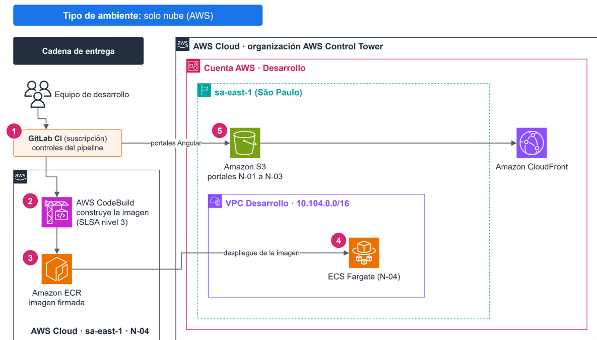
Figura 5 Ambiente de Desarrollo
