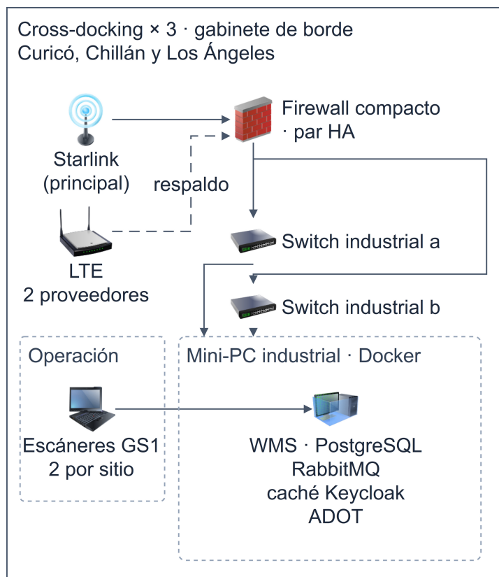
Figura 16 Gabinete de borde de las plataformas de cross-docking
