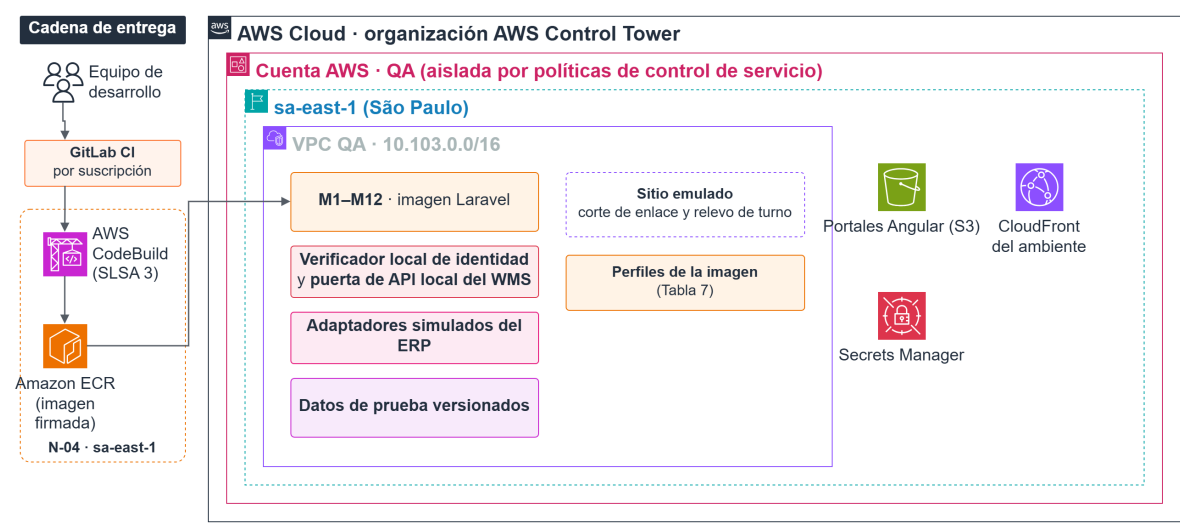
Figura 3 Ambiente de QA
