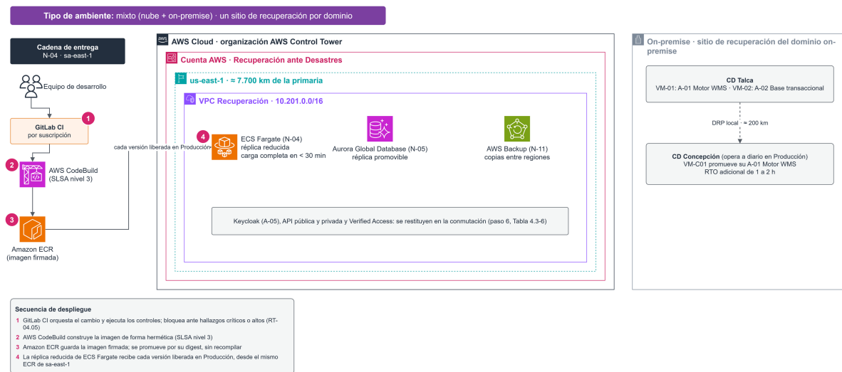
Figura 9 Ambiente de Recuperación ante Desastres
