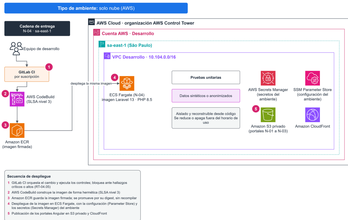
Figura 5 Ambiente de Desarrollo
