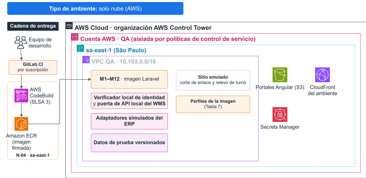
Figura 4 Ambiente de QA
