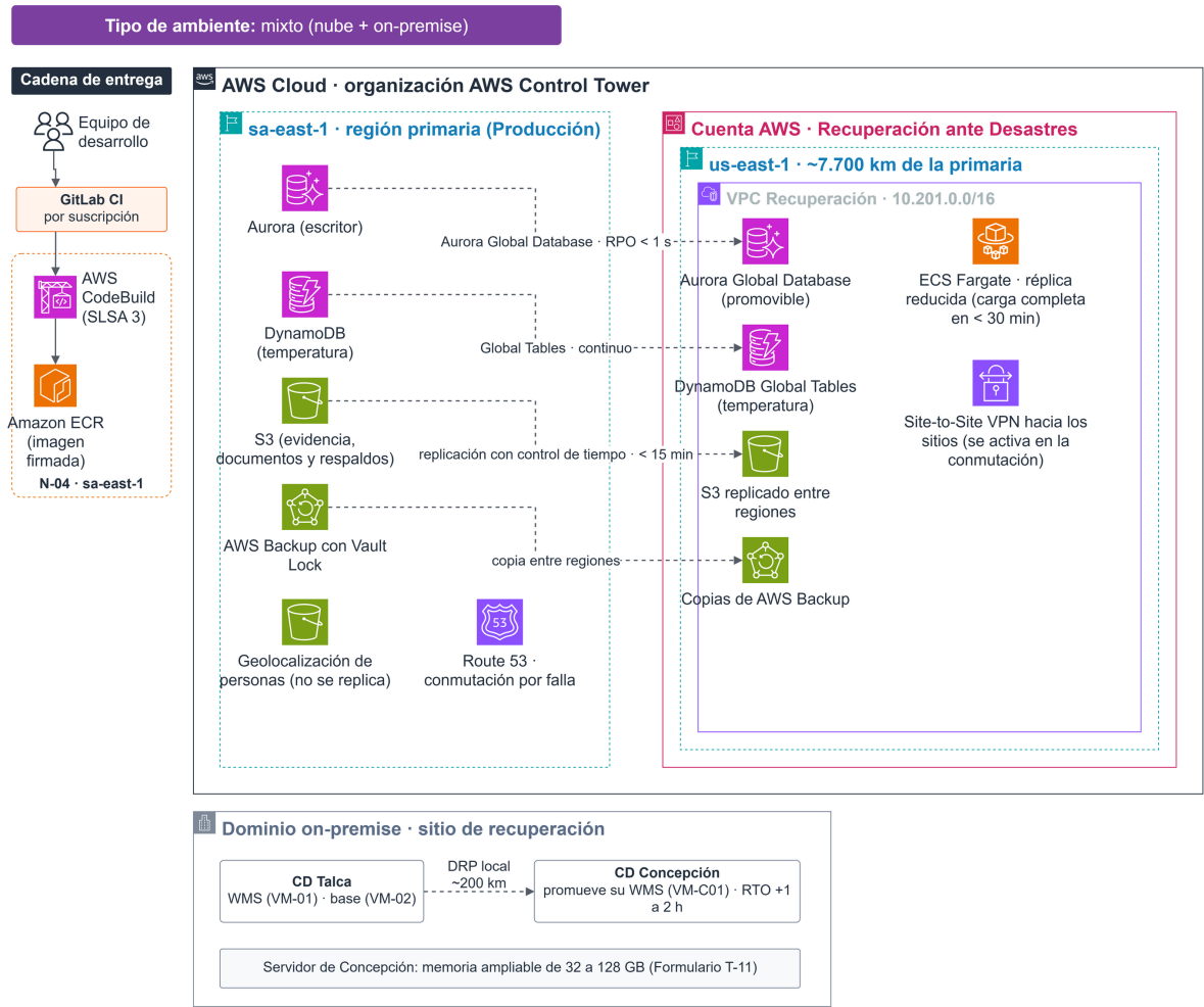
Figura 7 Ambiente de Recuperación ante Desastres
