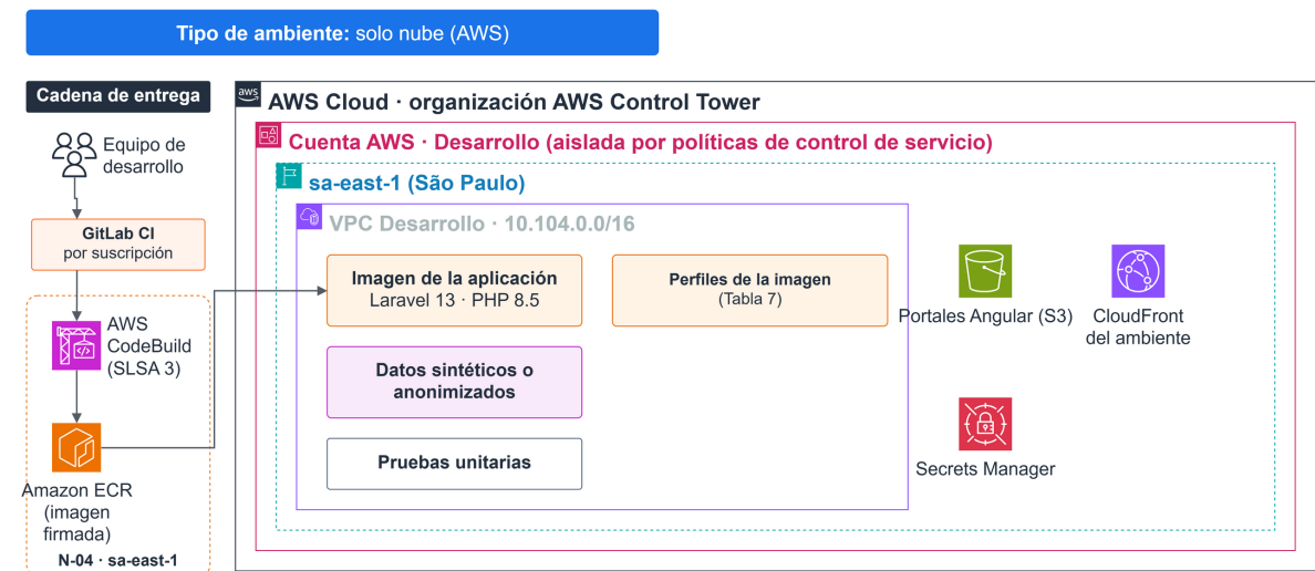
Figura 3 Ambiente de Desarrollo
