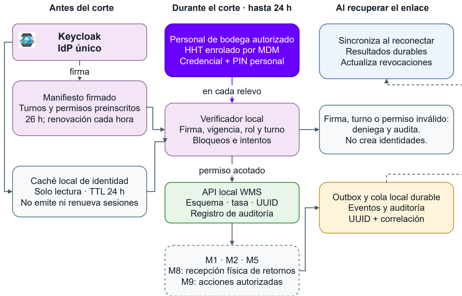
Figura 5 Identidad y puerta de API local durante un corte de 24 horas
