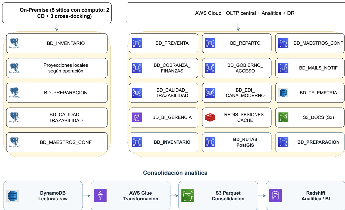
Figura 10 Datos: propiedad y persistencia híbrida
