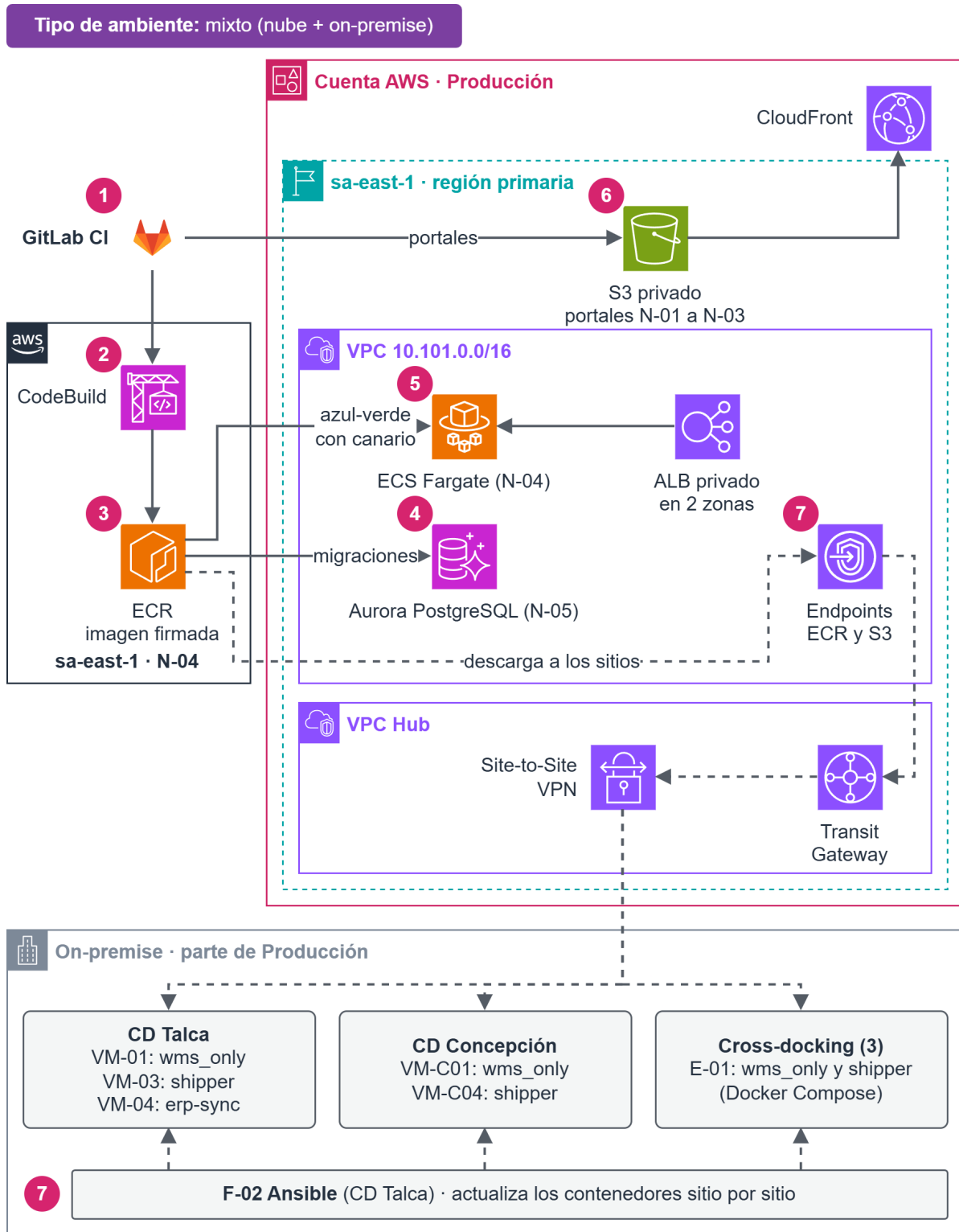
Figura 22 Ambiente de Producción
