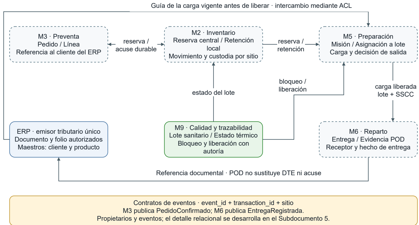
Figura 13 Dominio lógico: entidades, módulos responsables y eventos
