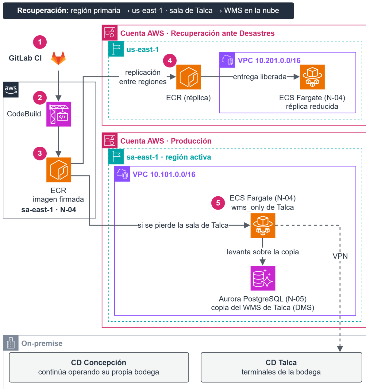
Figura 23 Ambiente de Recuperación ante Desastres
