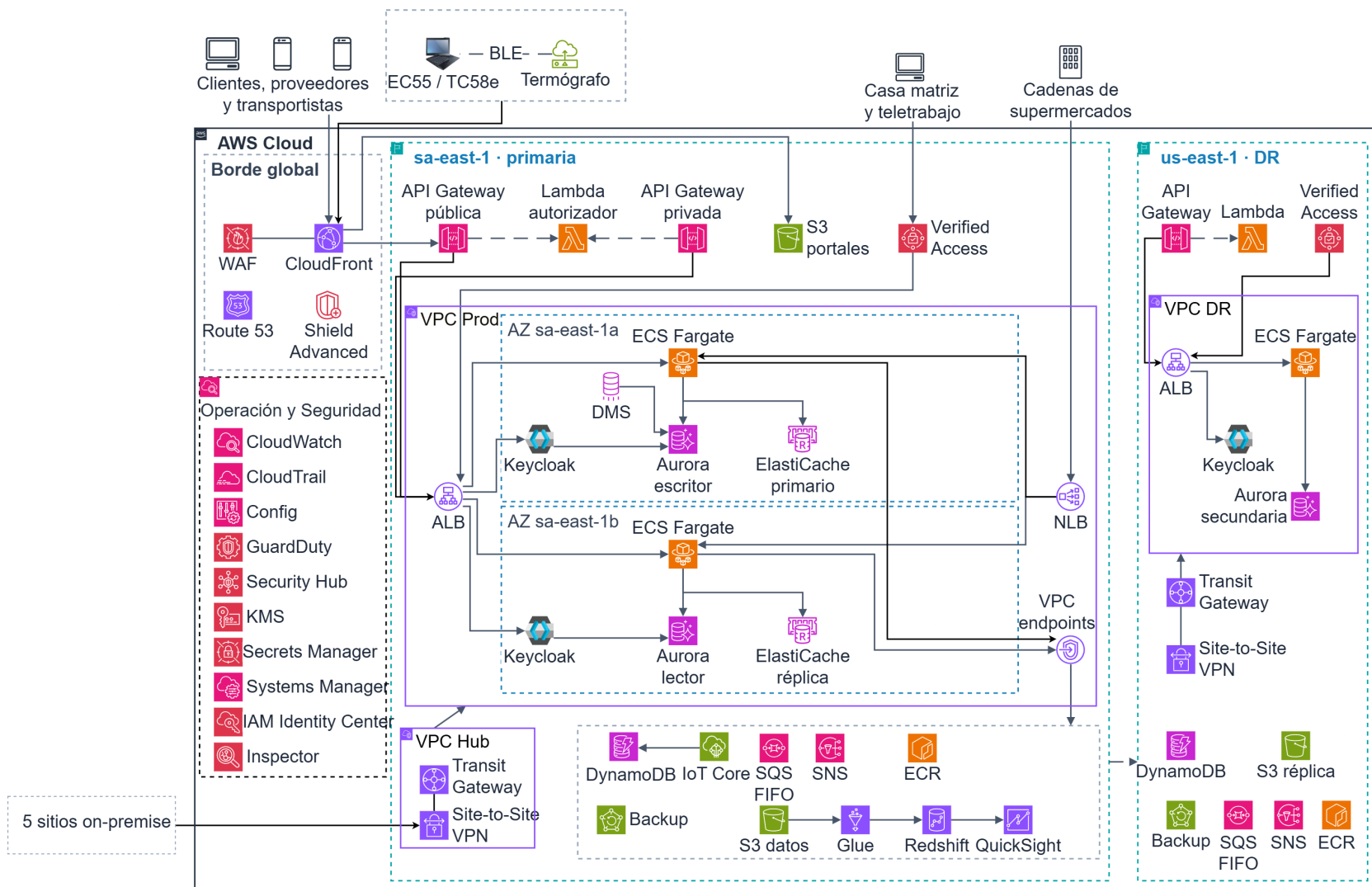
Figura 18 Topología de los servicios en AWS: región primaria sa-east-1 y región de recuperación us-east-1 Fuente: elaboración propia.
