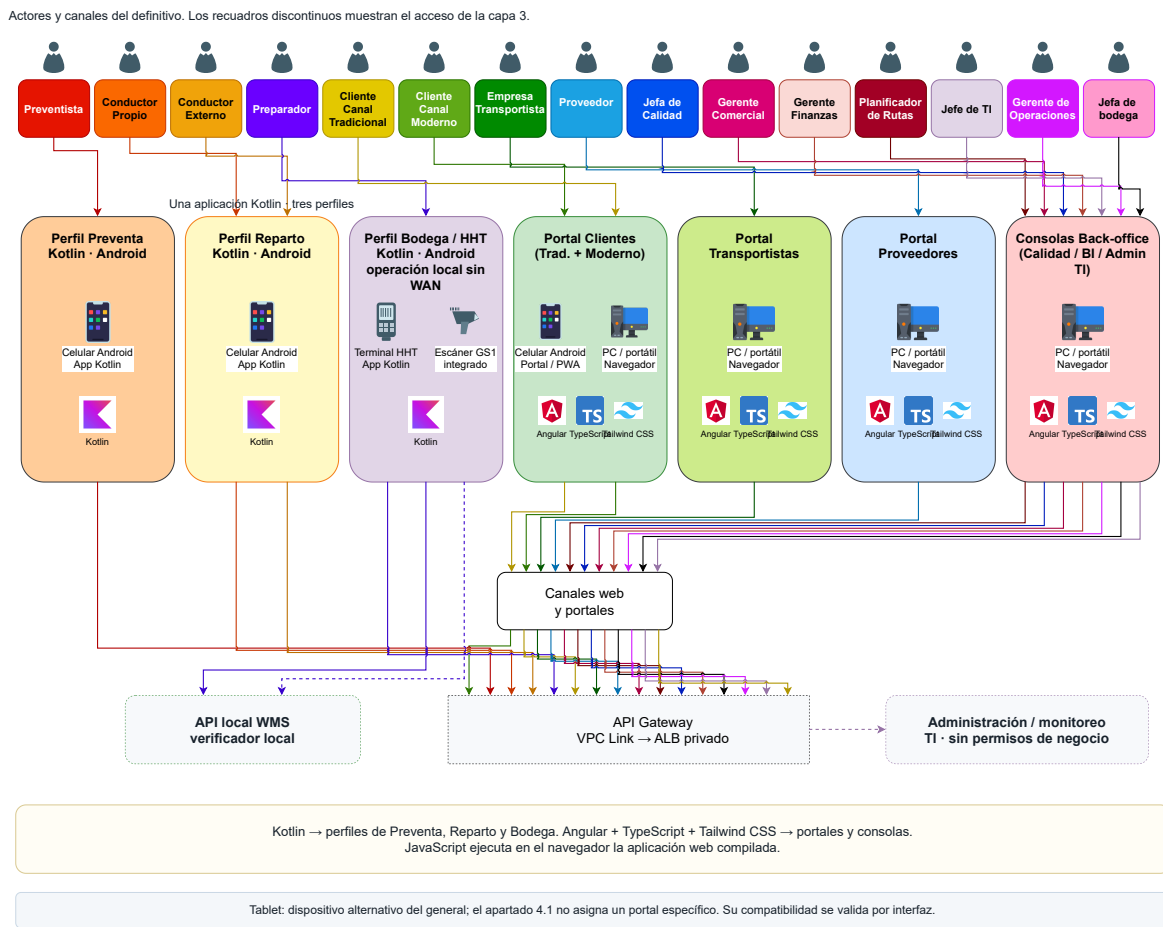
Figura 2 Presentación: aplicaciones y superficies de trabajo
