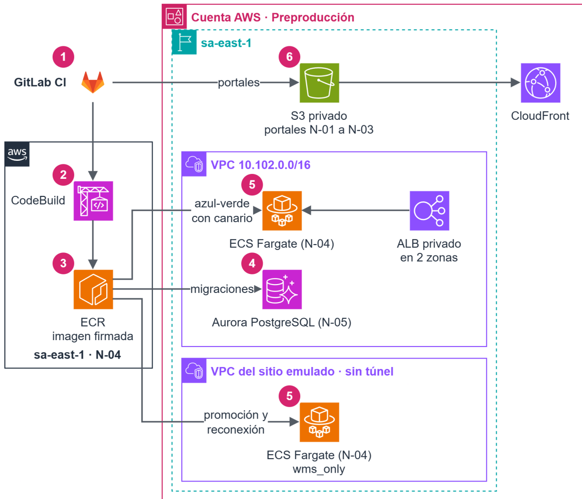
Figura 21 Ambiente de Preproducción
