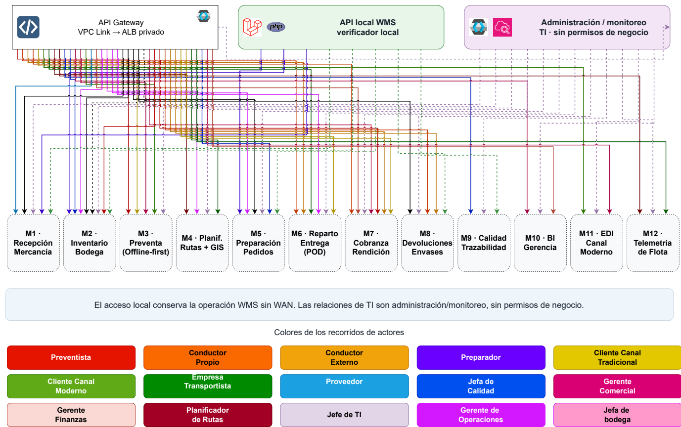
Figura 4 Puertas de servicio: recorrido central y local
