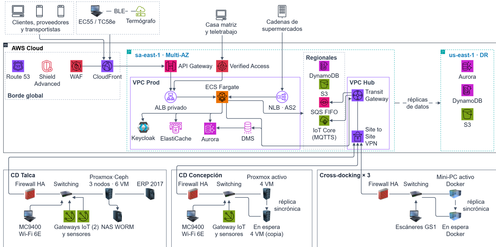
Figura 14 Vista general de la arquitectura física híbrida Fuente: elaboración propia.
