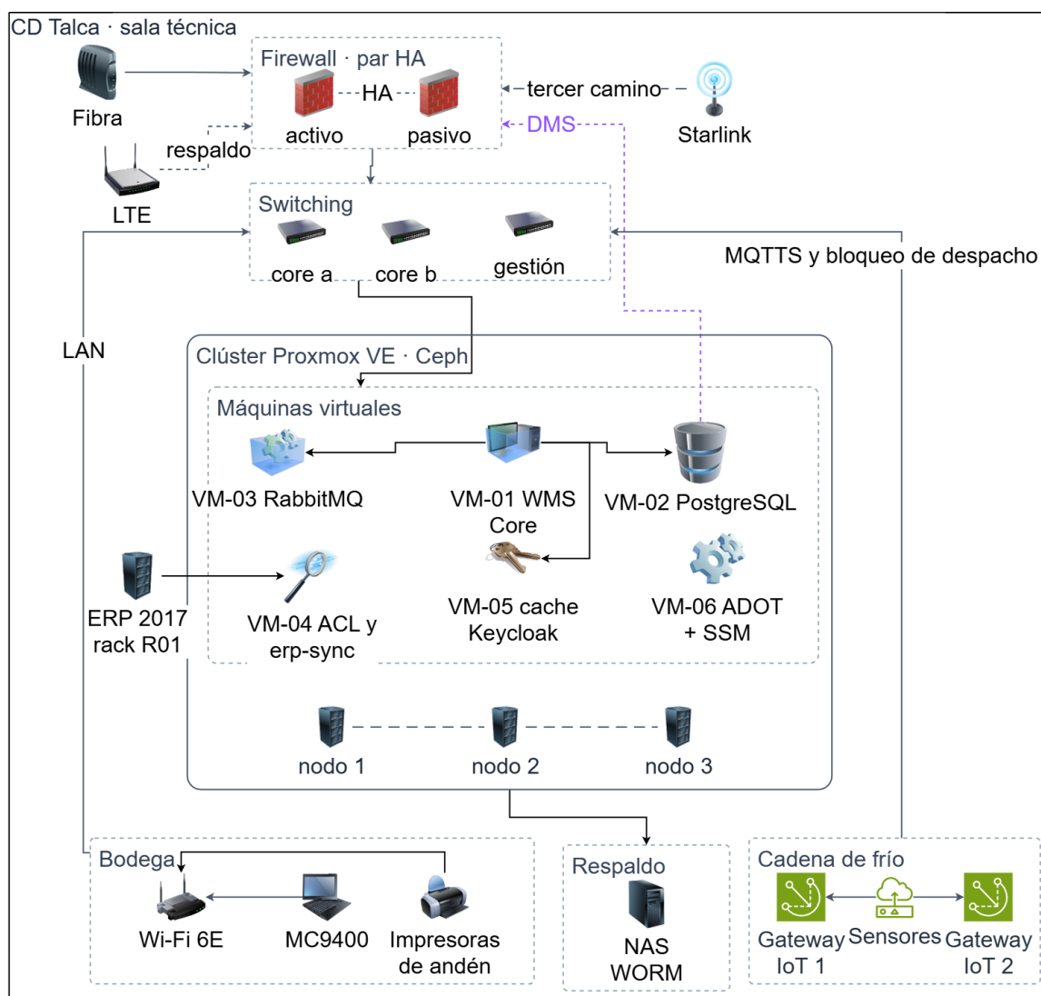
Figura 24 Arquitectura física del sitio on-premise del CD Talca
