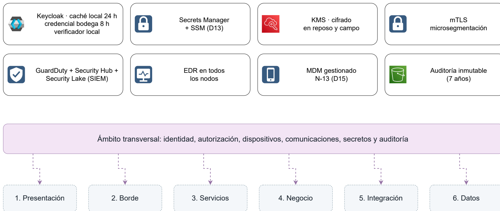
Figura 11 Seguridad: identidad y autorización transversal
