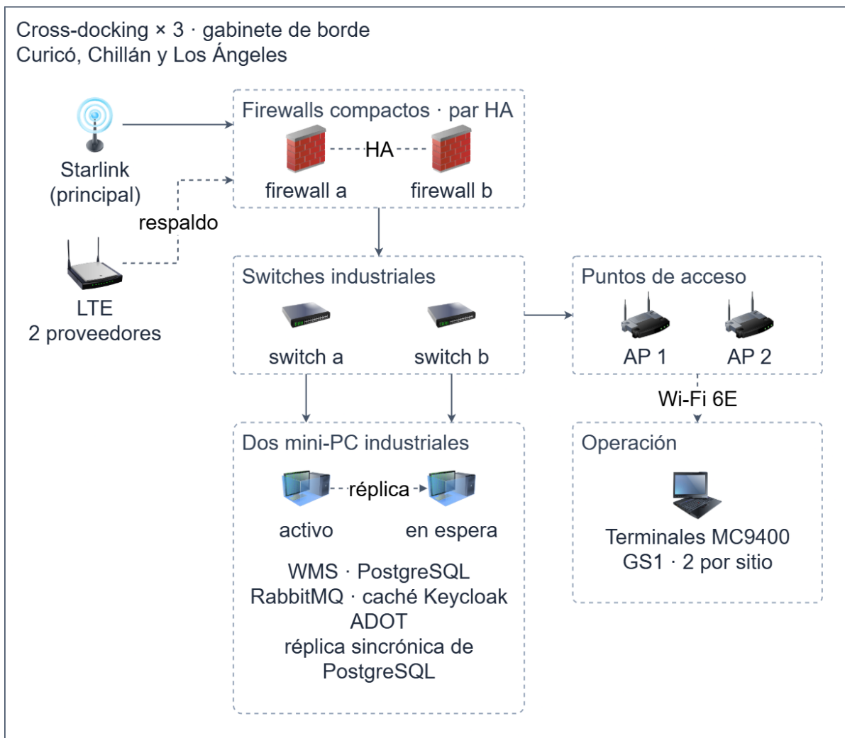
Figura 15 Gabinete de borde de las plataformas de cross-docking Fuente: elaboración propia.
