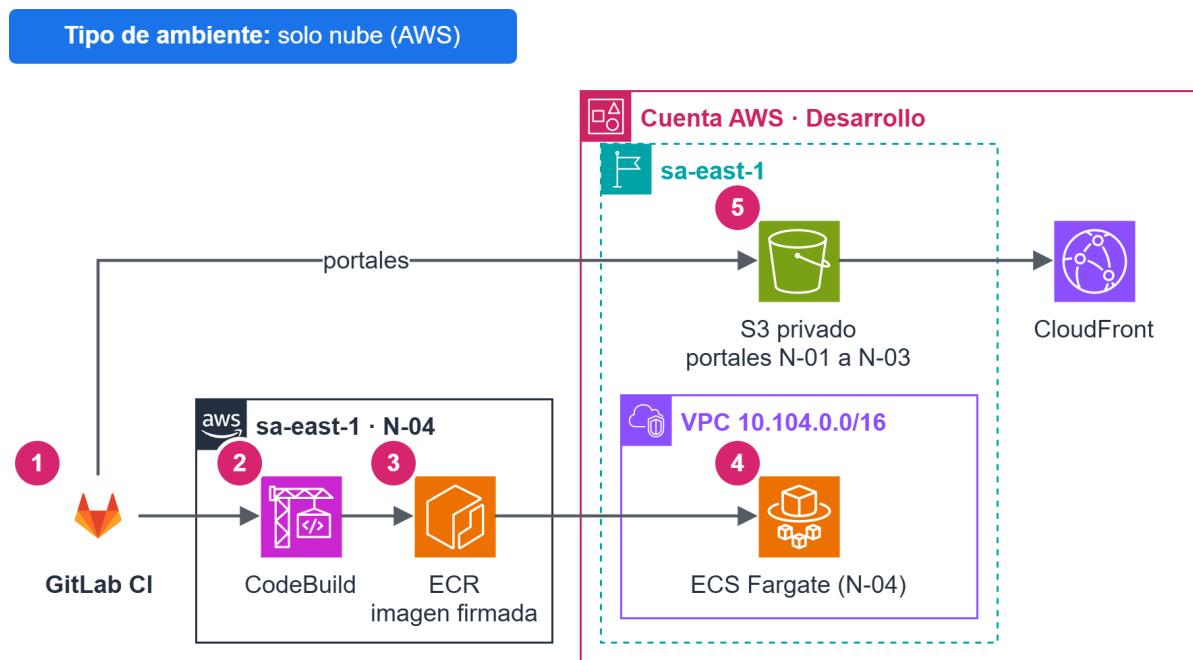
Figura 19 Ambiente de Desarrollo
