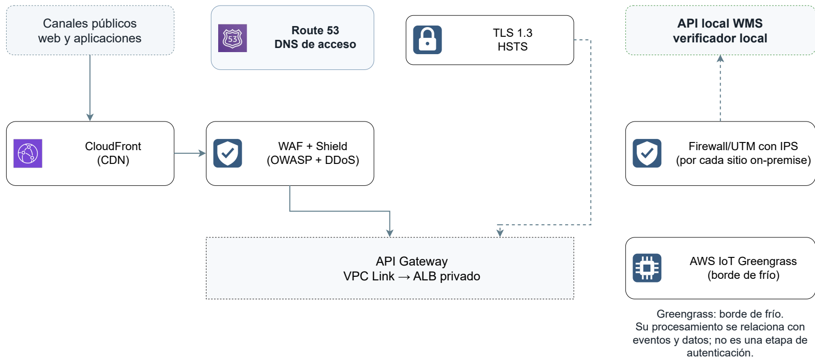
Figura 3 Borde: entradas públicas, privadas y locales
