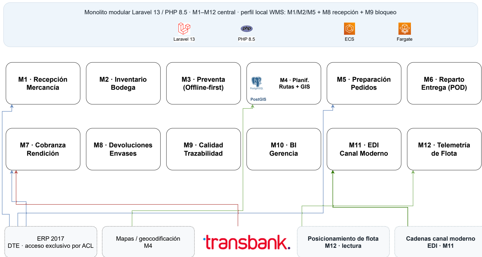
Figura 6 Negocio: monolito modular Laravel y sus doce módulos
