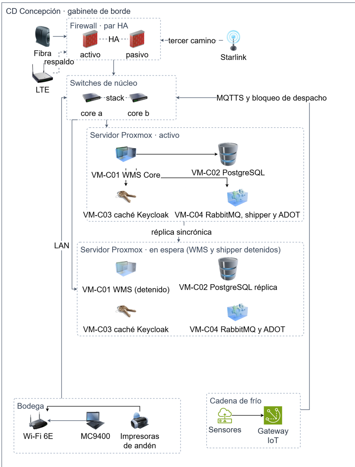
Figura 16 Gabinete de borde del CD Concepción
