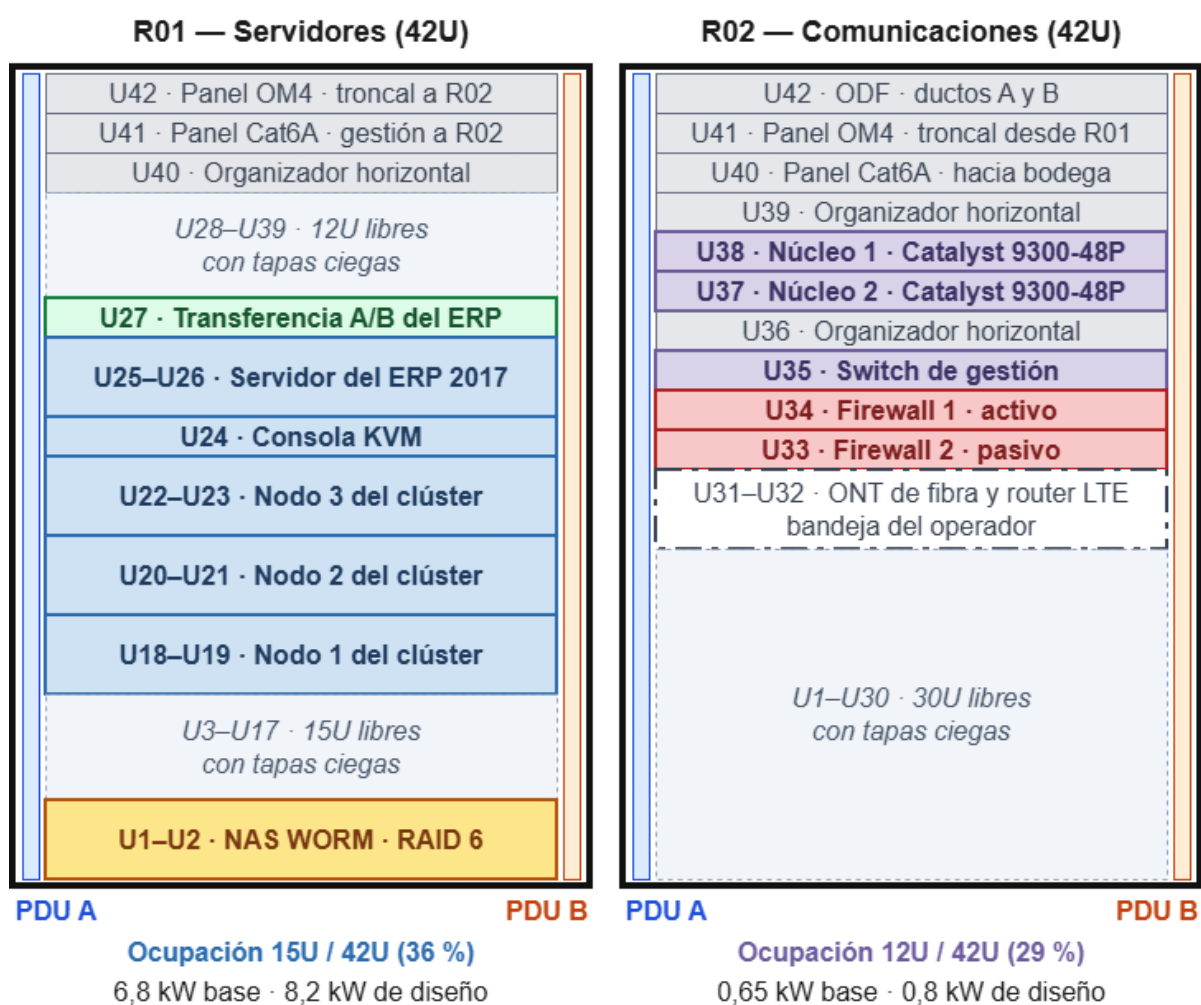
Figura 25 Distribución de U y ocupación proyectada de los racks del CD Talca Fuente: elaboración propia.
