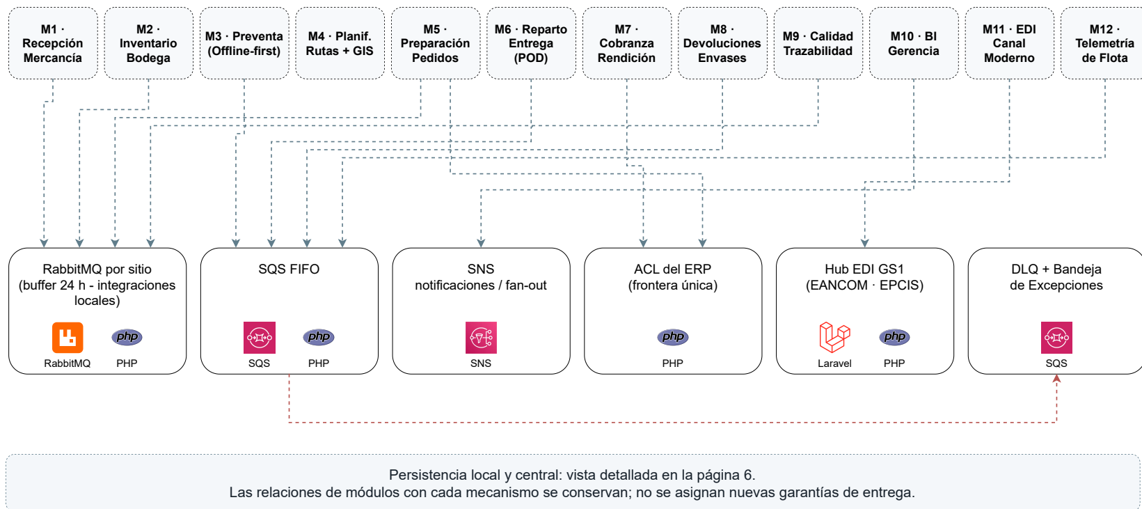
Figura 7 Integración: continuidad local y contratos con terceros
