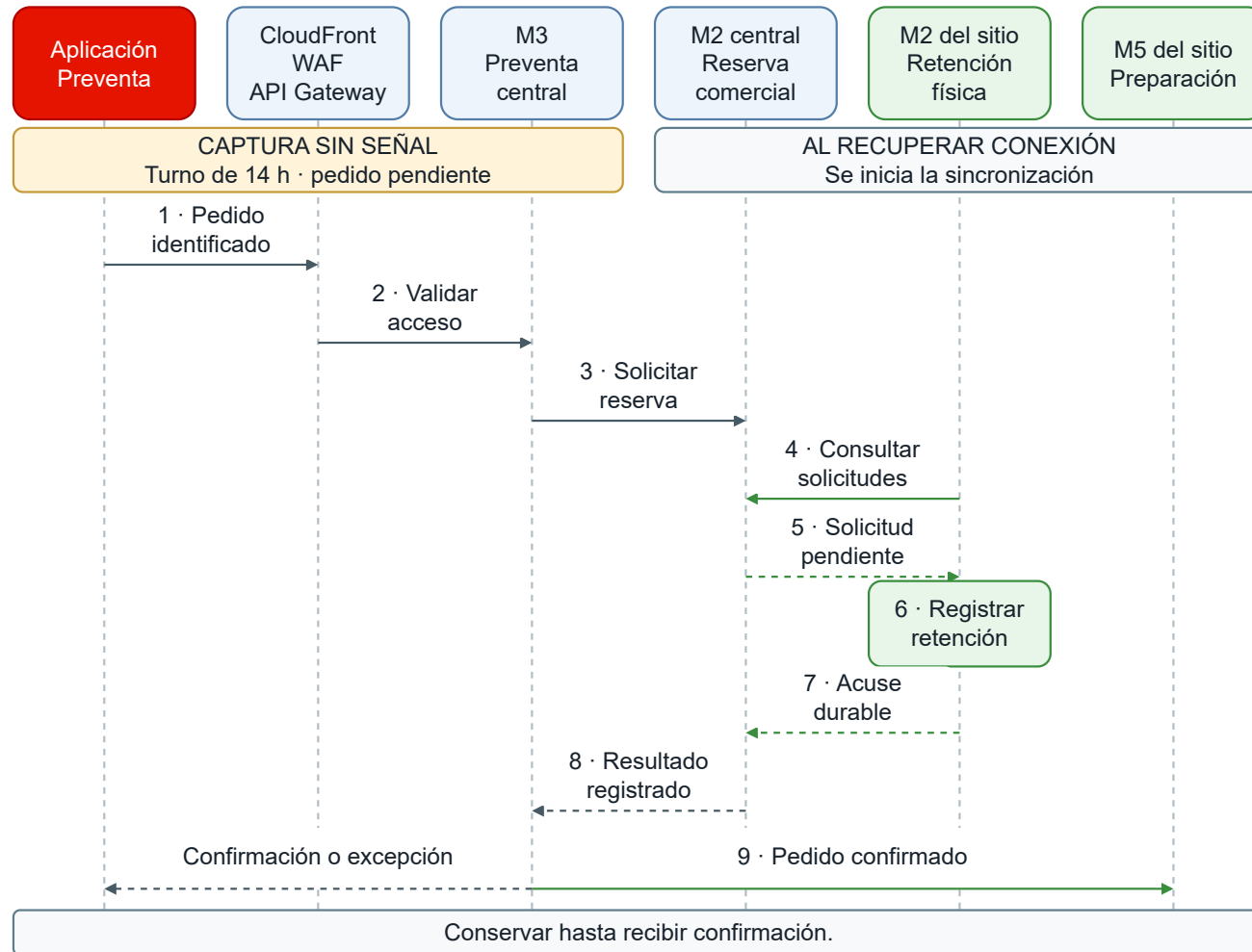
Figura 9 Secuencia lógica del pedido capturado sin conexión
