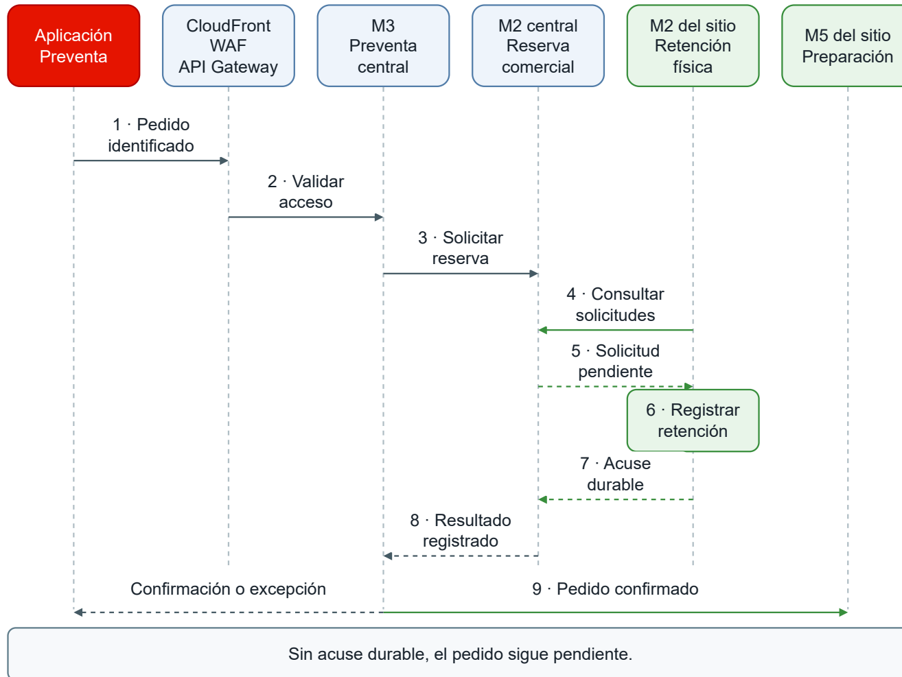
Figura 8 Secuencia lógica del pedido con conexión
