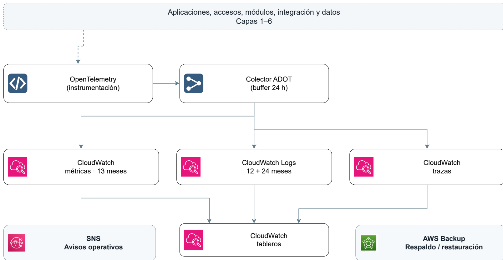
Figura 12 Observabilidad: correlación de nube y sitios
