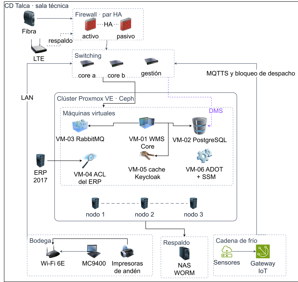
Figura 1 Arquitectura física del sitio on-premise del CD Talca Fuente: elaboración propia.
