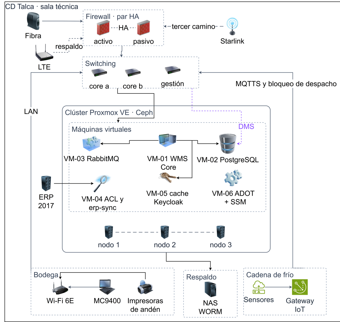
Figura 27 Arquitectura física del sitio on-premise del CD Talca
