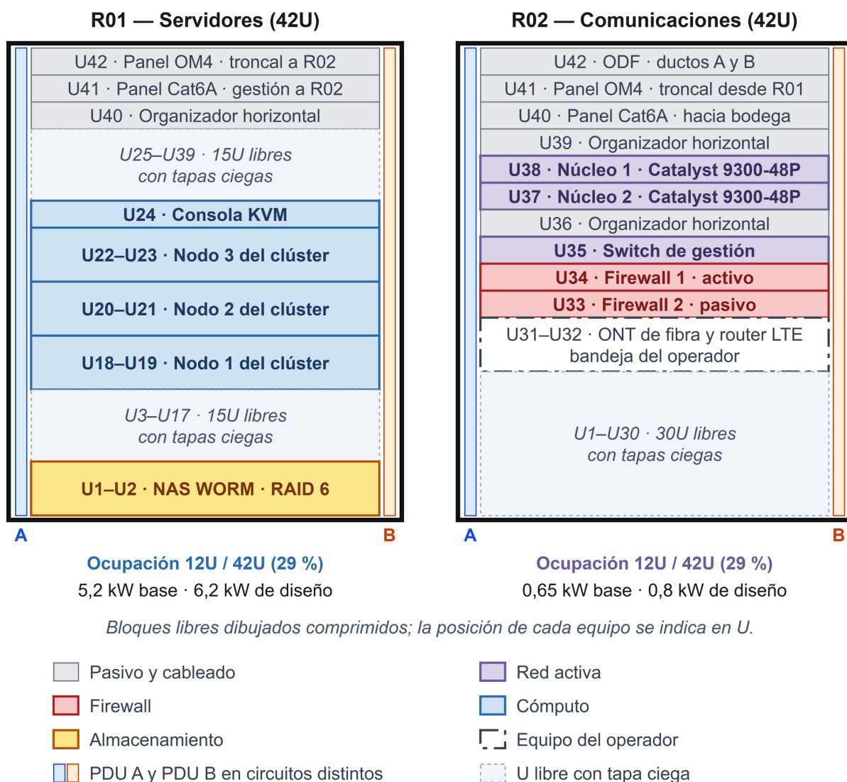
Figura 28 Distribución de U y ocupación proyectada de los racks del CD Talca
