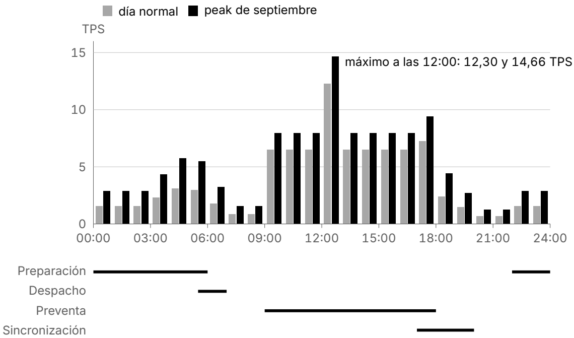
Figura 9 Tasas totales por hora en régimen normal y en septiembre.
