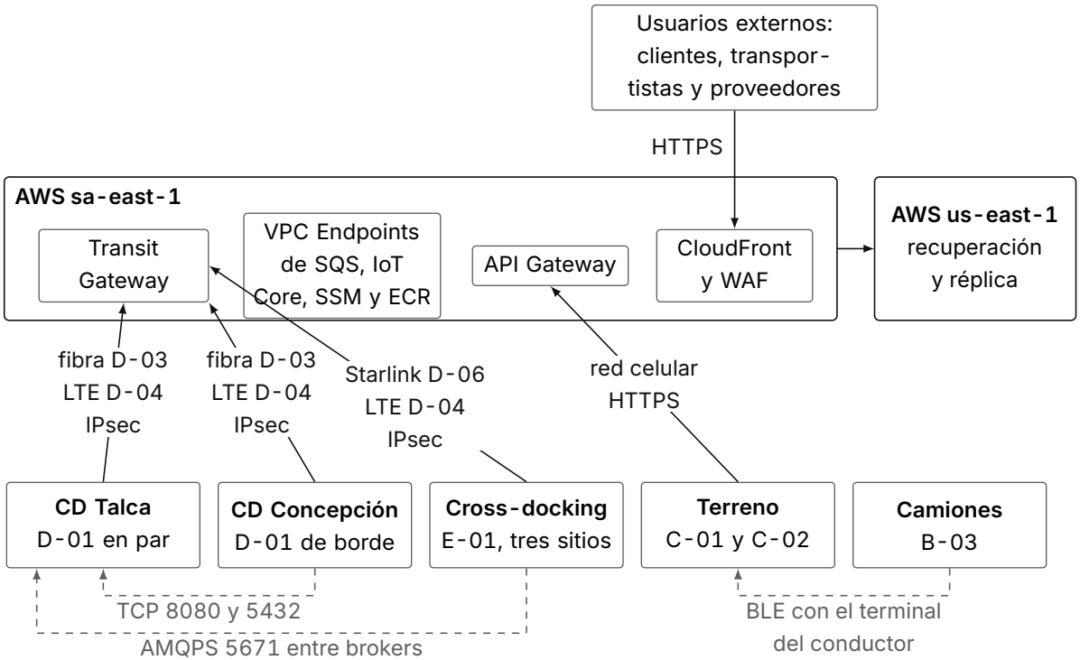
Figura 7 Conexiones entre los sitios, el terreno y la nube
