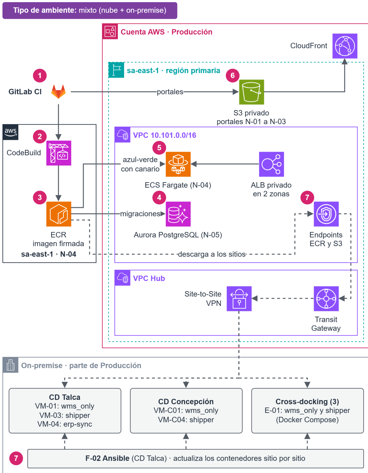
Figura 23 Ambiente de Producción
