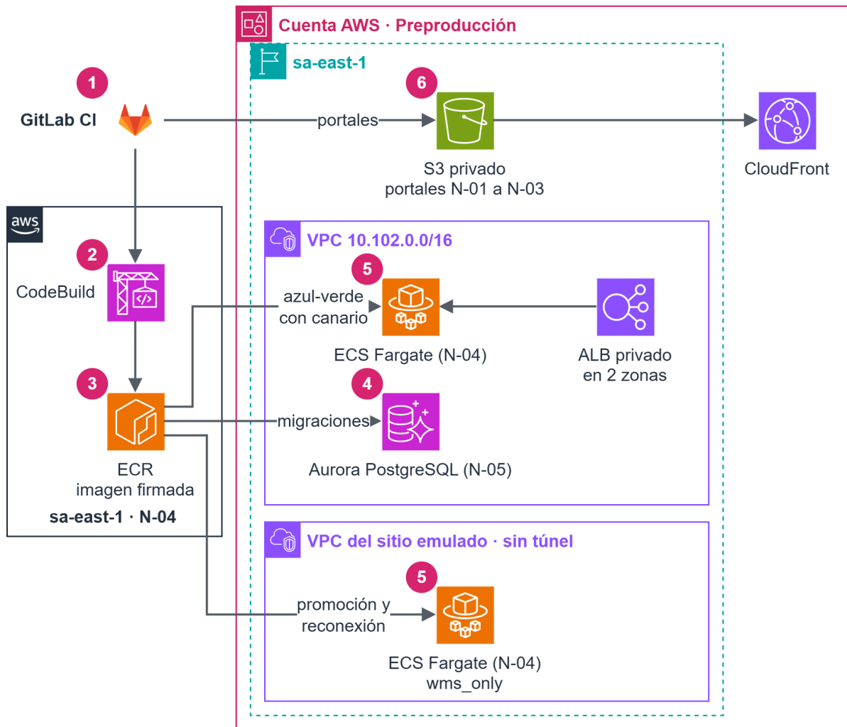
Figura 22 Ambiente de Preproducción
