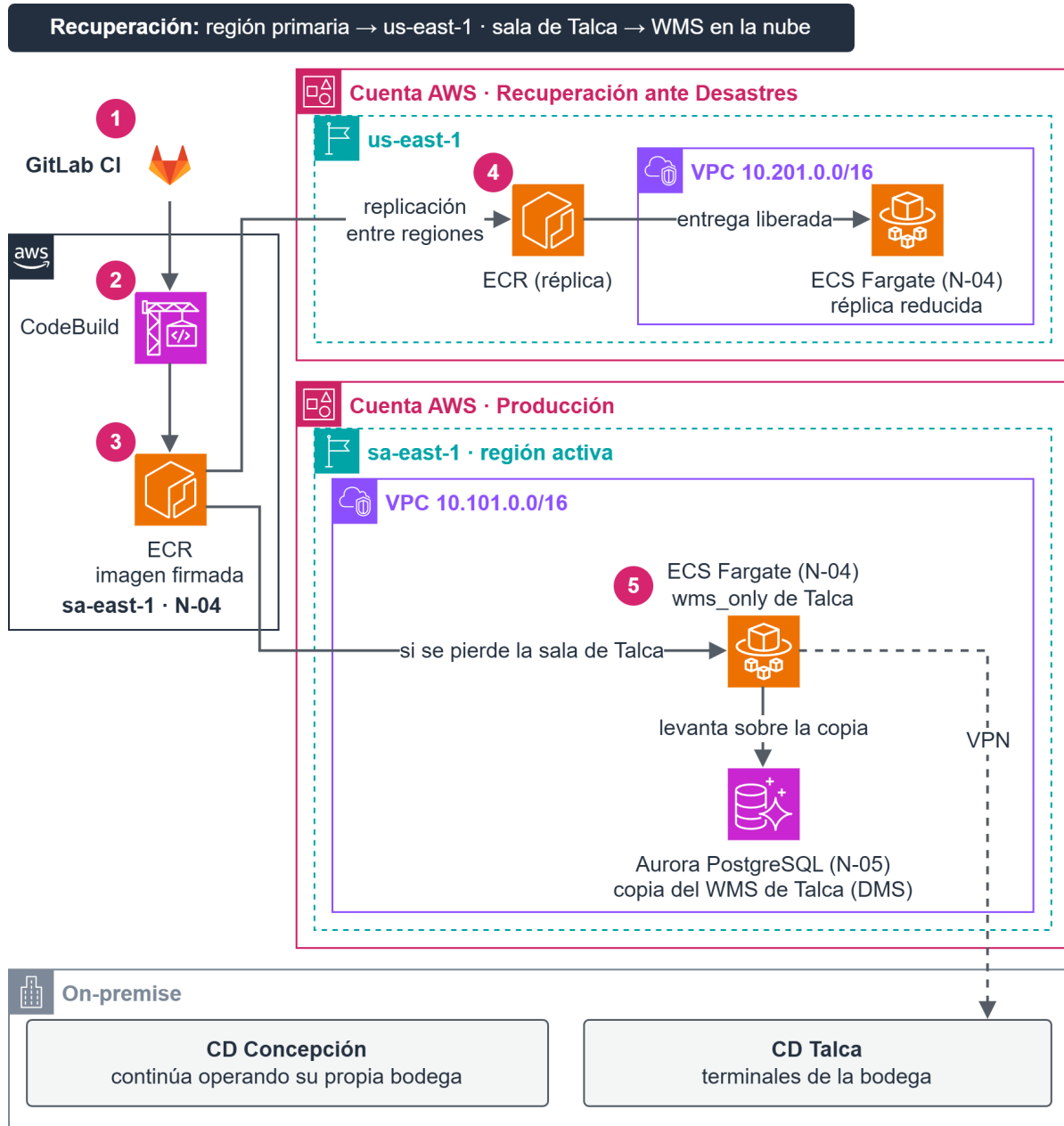
Figura 24 Ambiente de Recuperación ante Desastres
