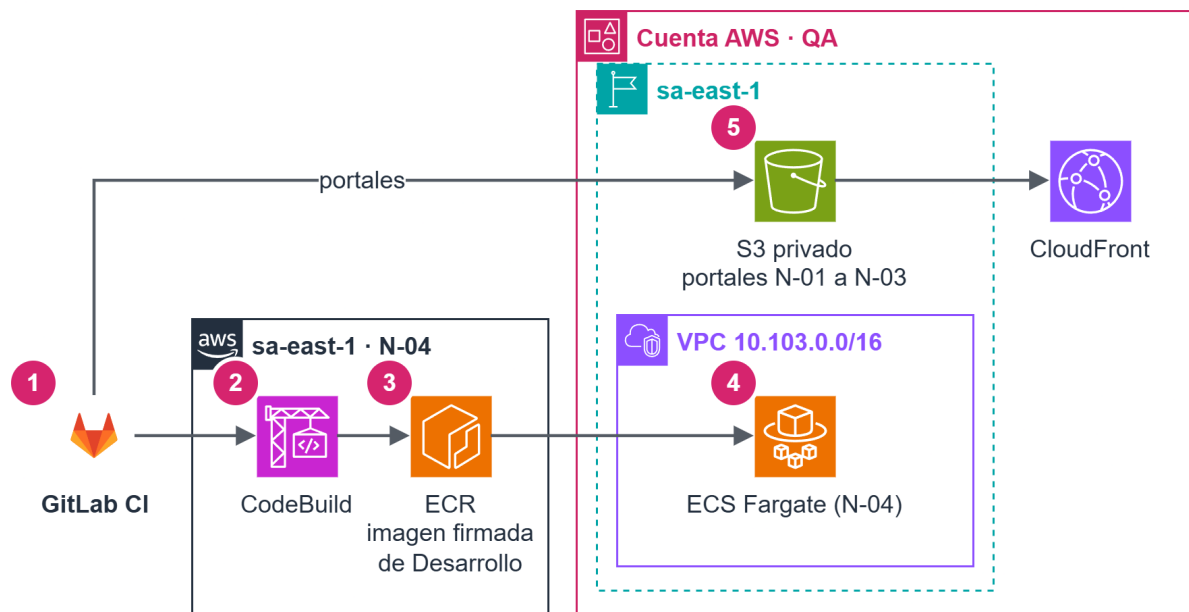
Figura 21 Ambiente de QA
