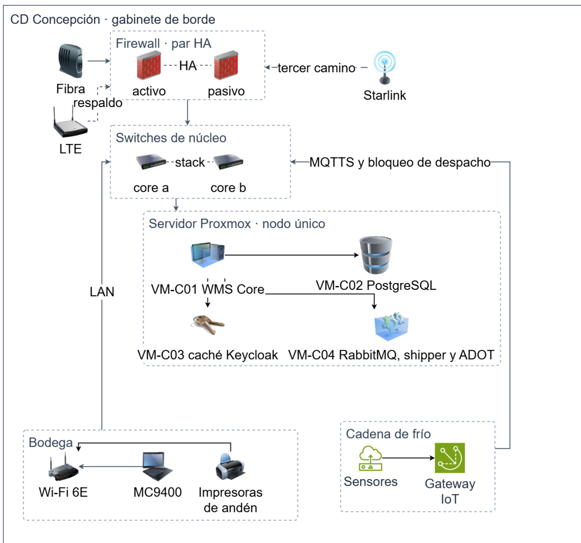
Figura 17 Gabinete de borde del CD Concepción
