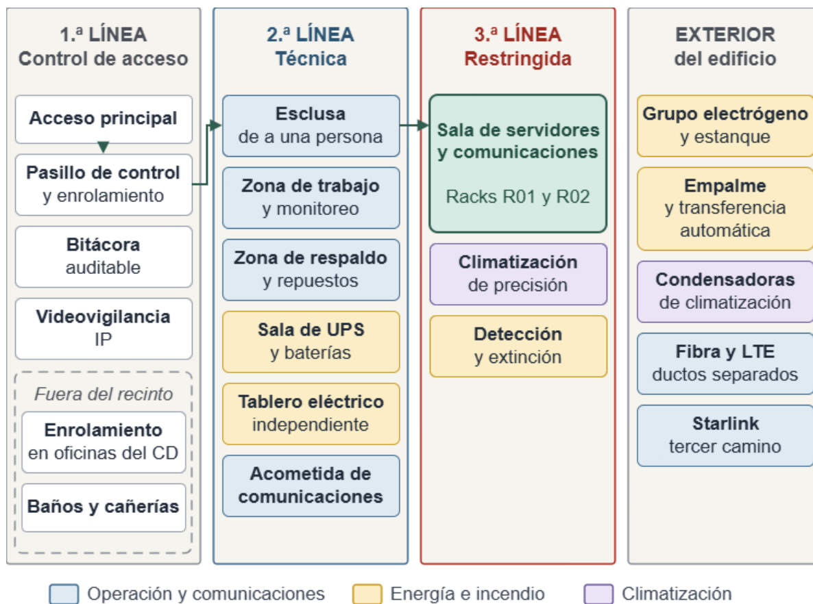
Figura 27 Esquema de zonas y líneas de acceso del recinto técnico del CD Talca
