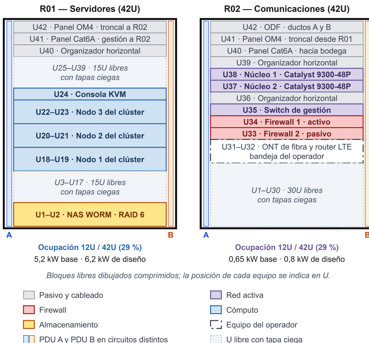
Figura 26 Distribución de U y ocupación proyectada de los racks del CD Talca
