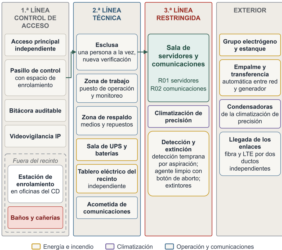
Figura 27 Distribución interna del recinto técnico del CD Talca por zonas y líneas de acceso
