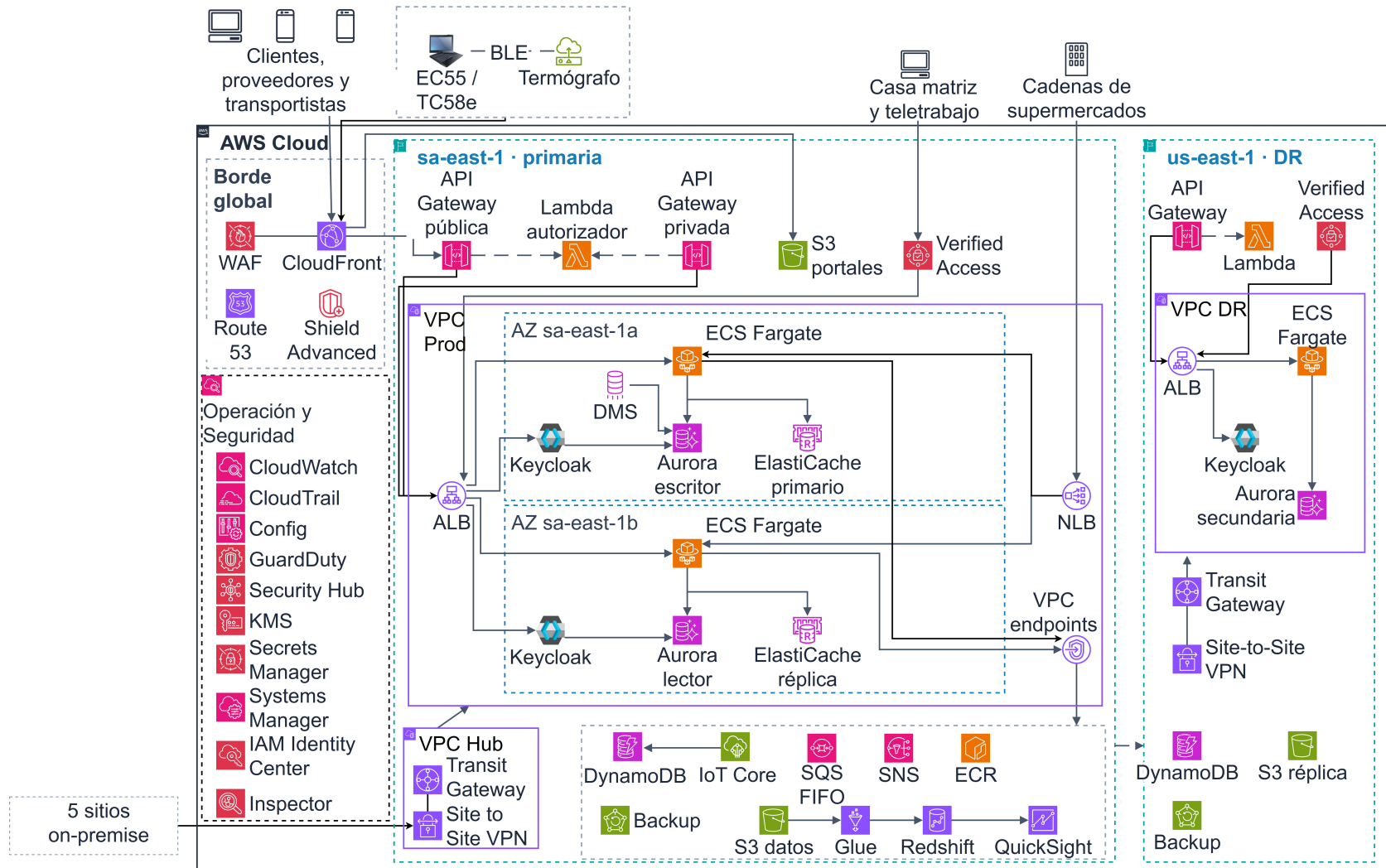
Figura 19 Topología de los servicios en AWS: región primaria sa-east-1 y región de recuperación us-east-1
