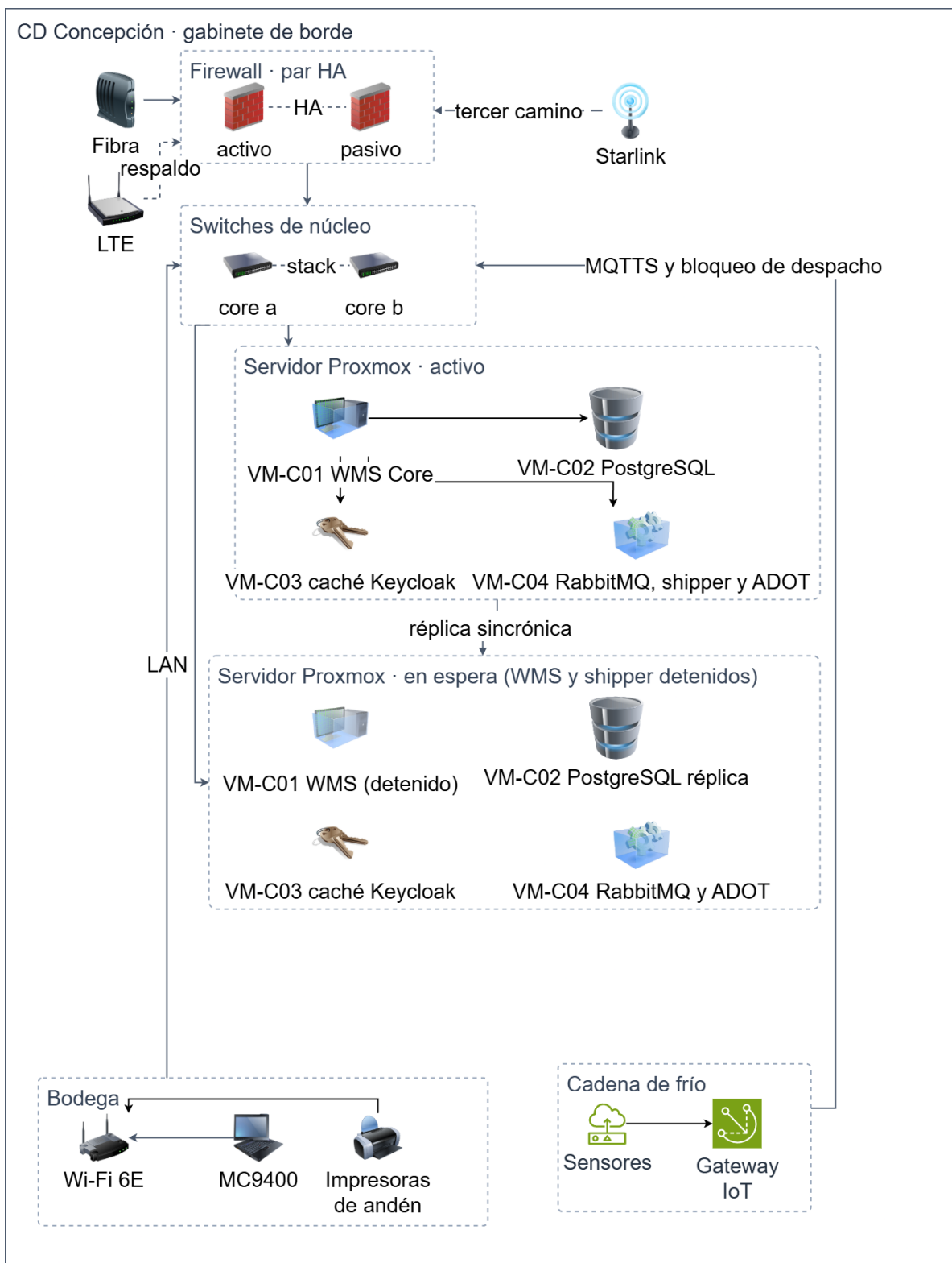
Figura 17 Gabinete de borde del CD Concepción
