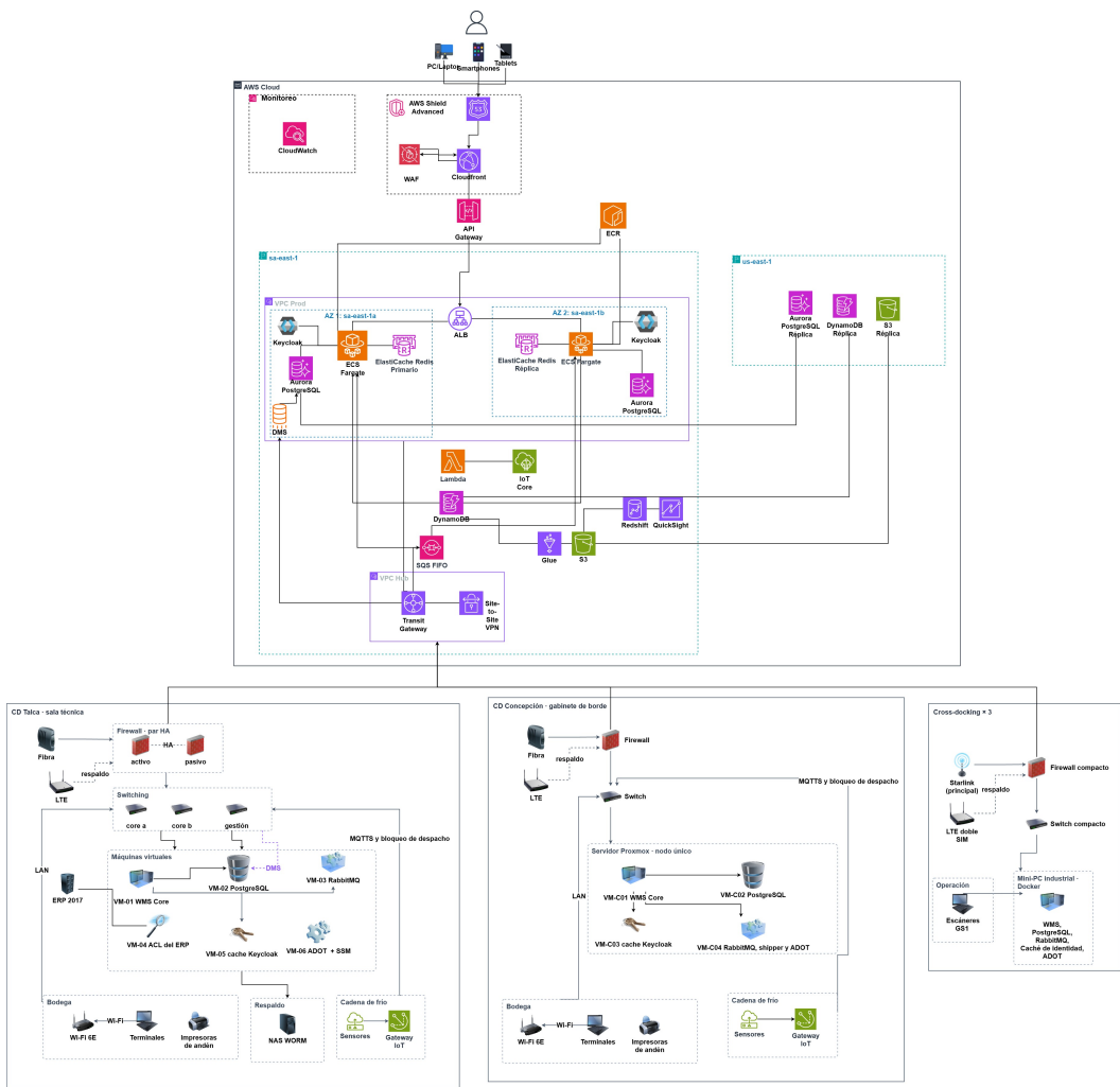
Figura 1 Vista general de la arquitectura física híbrida
