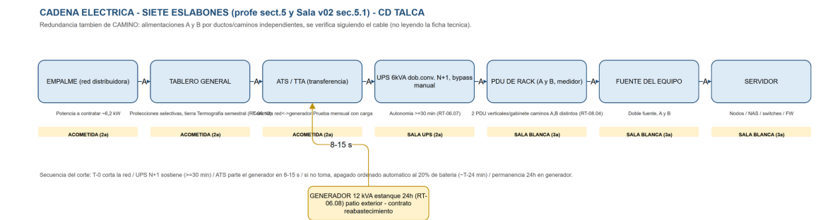
Figura 3 Cadena eléctrica del recinto: acometida, transferencia automática, generación autónoma, alimentación ininterrumpida y distribución A/B por gabinete
