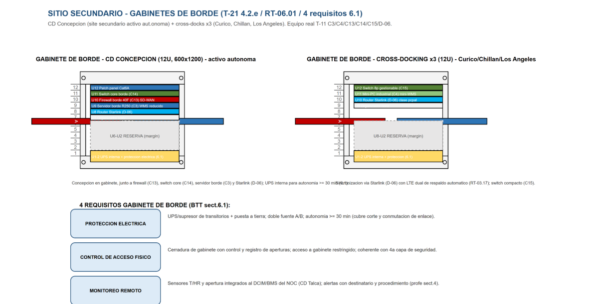
Figura 5 Gabinete de borde industrializado del CD Concepción y de las tres plataformas de cross-docking: alimentación protegida, control de acceso y monitoreo remoto dimensionados al sitio (numeral 6.1, tipología de borde operacional)
