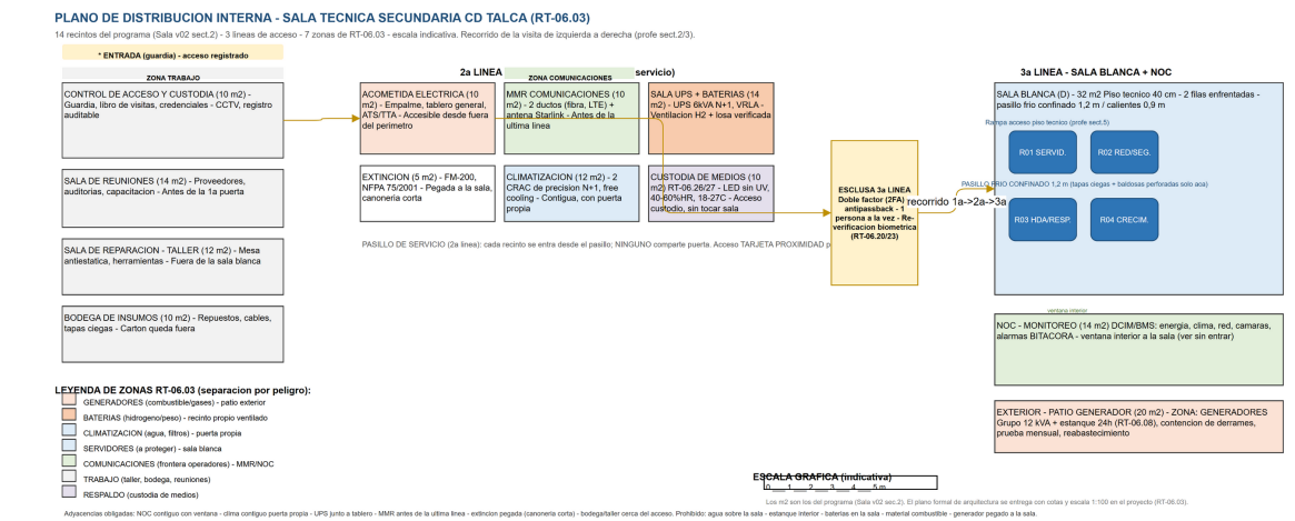
Figura 2 Plano de distribución interna del recinto técnico, con la separación de las zonas de generador, baterías, climatización, servidores, comunicaciones y custodia de medios
