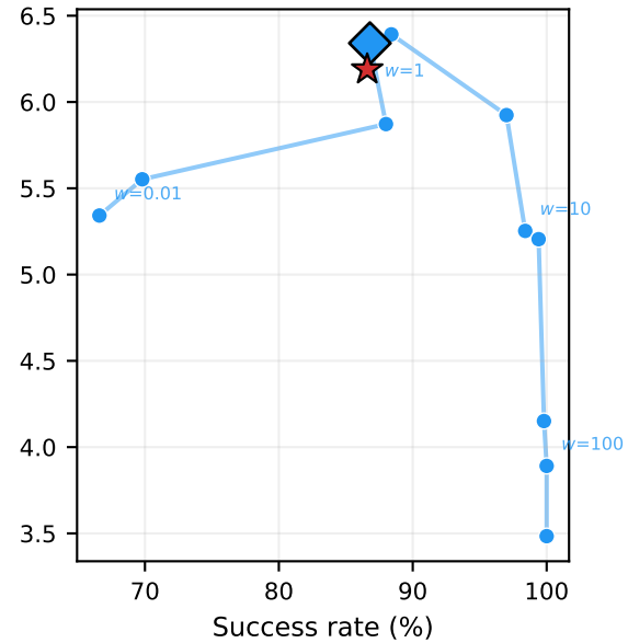
(d) Bandit
