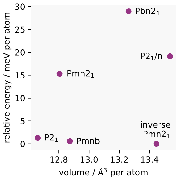
(b) \text{FeSiO}_4
