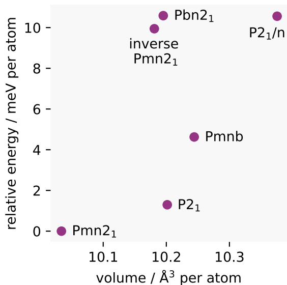
(a) \text{Li}_2\text{FeSiO}_4
