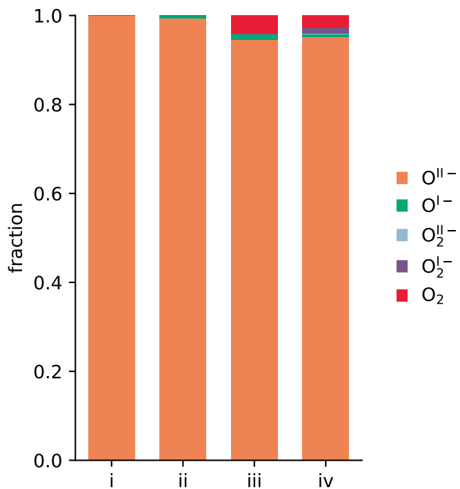
(d) 1000 K
