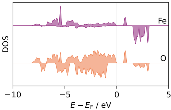
(c) \text{FeSiO}_4
