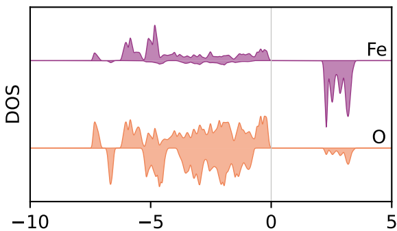
(b) \text{LiFeSiO}_4
