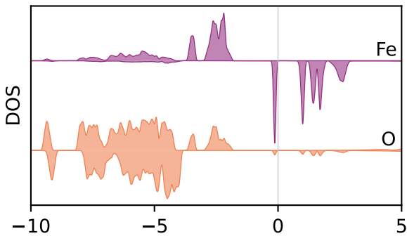
(a) \text{Li}_2\text{FeSiO}_4
