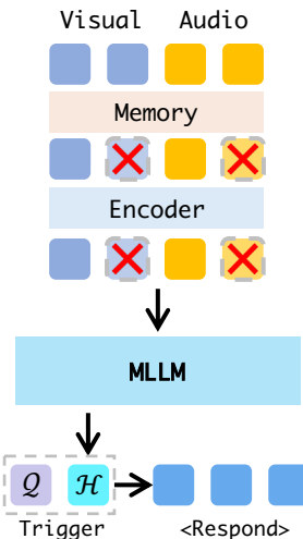
(D) StreamOV
