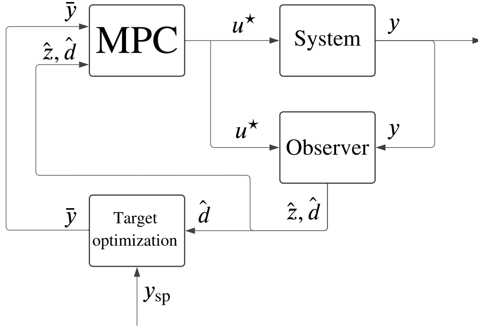
Figure 1: Closed-loop control structure. TODO: prerobiť tak aby znormalizoval fonty a haty, rozdeliť d a z
