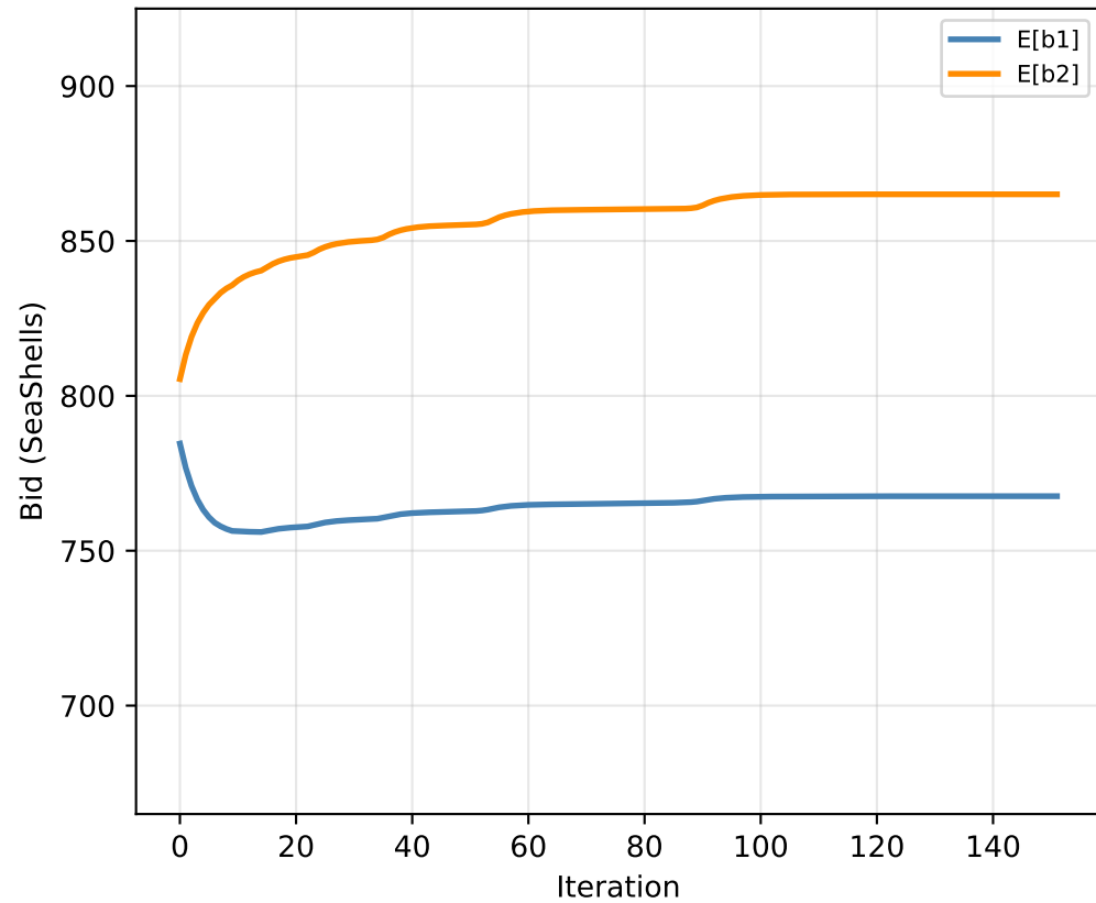
QRE
