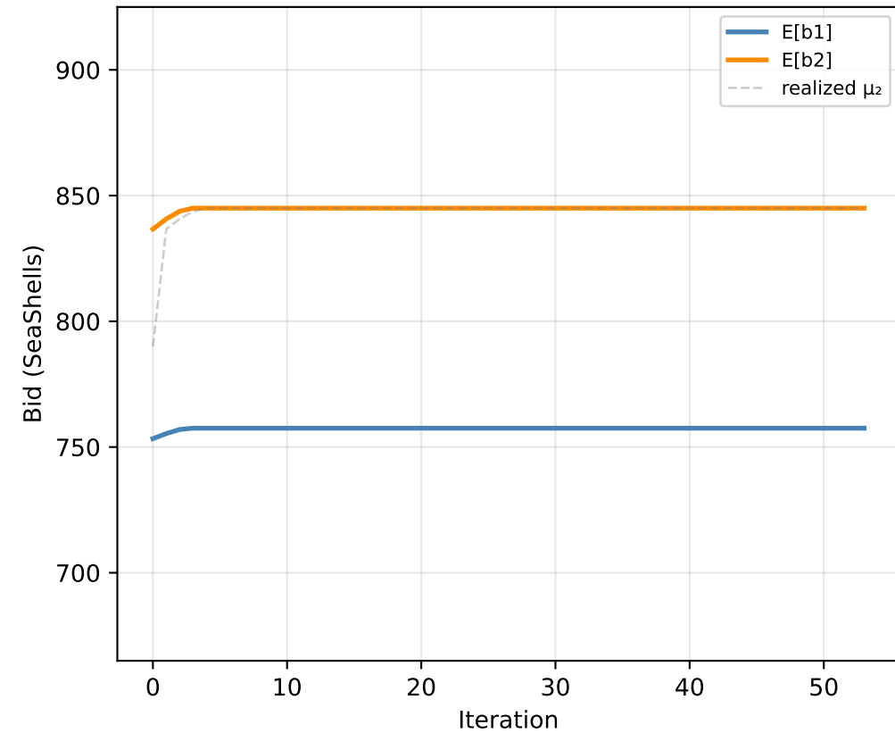
Monte Carlo
