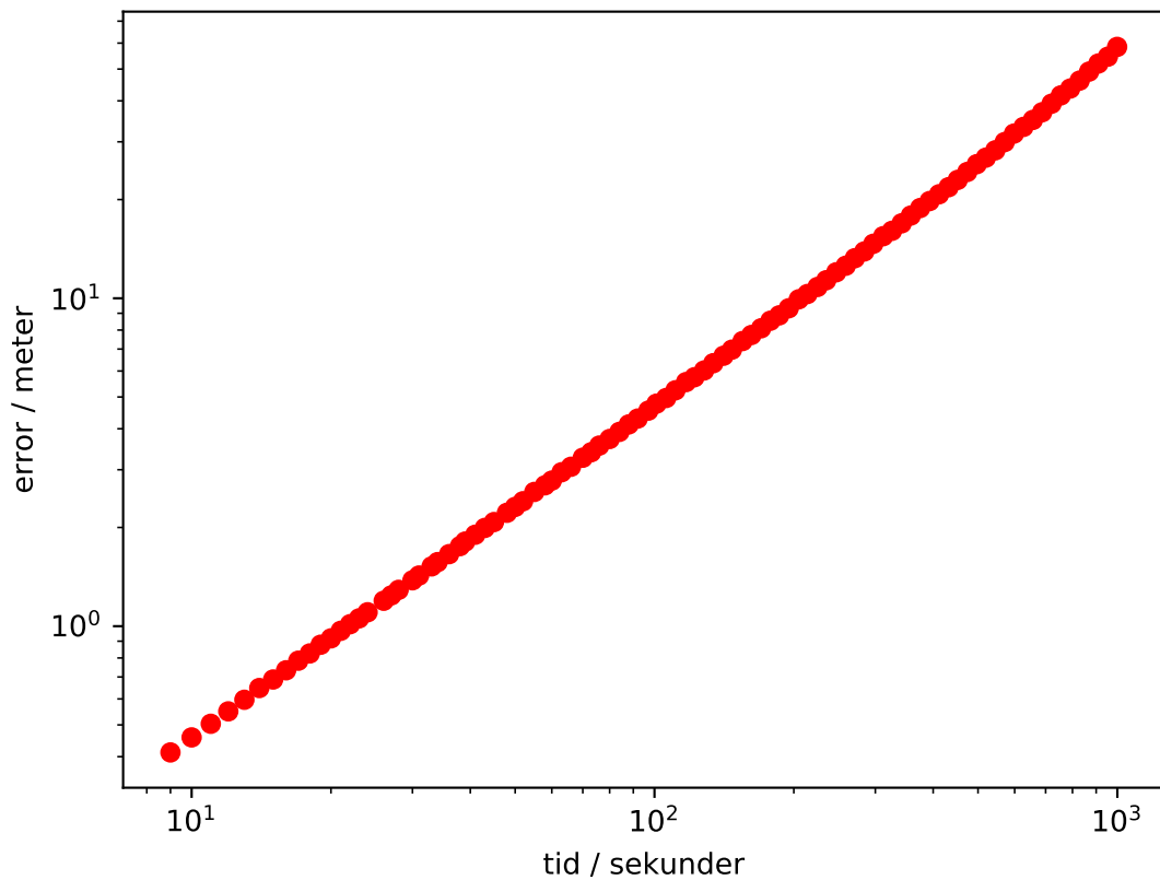
Global error
