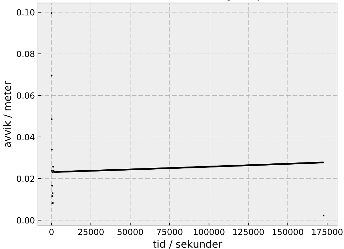
Avvik mellom Euler og Trapes
